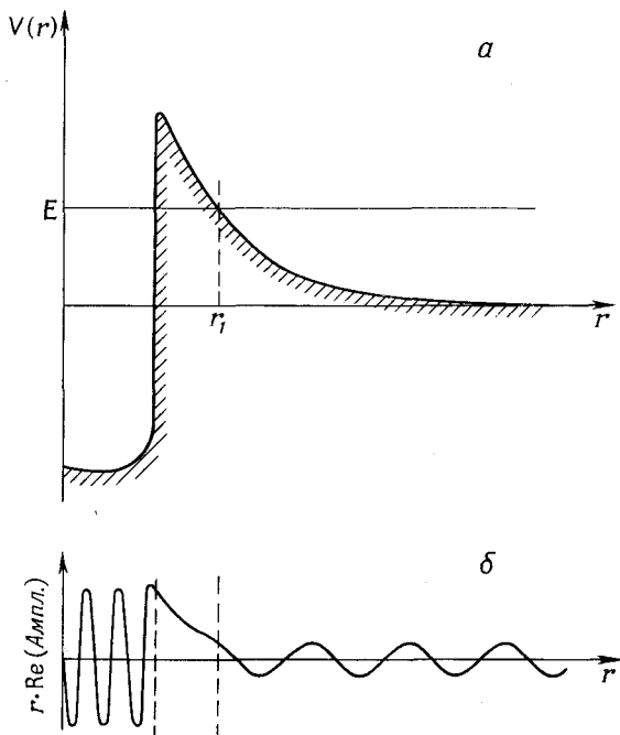
Ф и г. 5.б. Потенциал \alpha -частицы в ядре урана (а) и качественный вид амплитуды вероятности (б).
