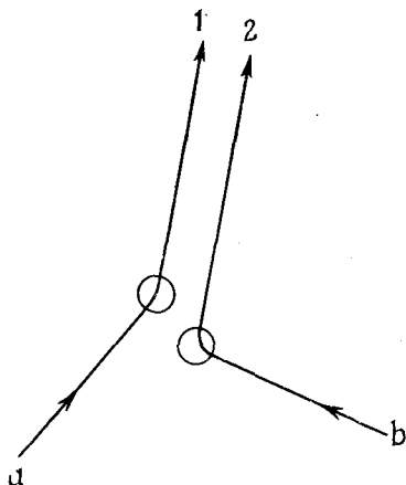
Ф и г . 2.3. Двойное рассеяние в близкие конечные состояния.
