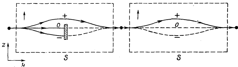
Фиг. 3.4. «Усовершенствованный» прибор Штерна—Герлаха в качестве фильтра.
