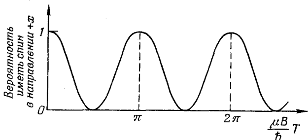
Ф и г. 5.10. Временная зависимость вероятности того, что частица со спином 1/2 окажется в состоянии (+) по отношению оси x .
