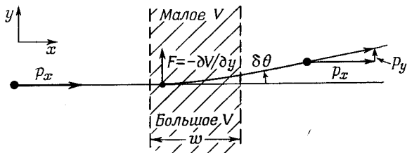
Фиг. 5.7. Отклонение частицы поперечным градиентом потенциала.
