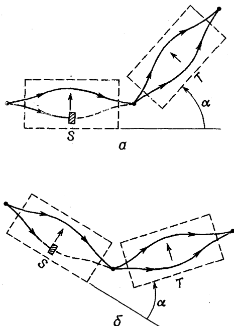
Ф и г. 4.2. Два эквивалентных эксперимента.
