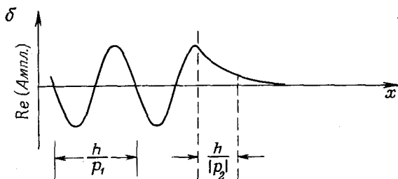
Фиг. 5.4. Амплитуда для частицы, приближающейся к сильно отталкивающему потенциалу.
