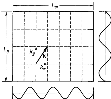
Фиг. 2.9. Типы стоячих волн в двух измерениях.
