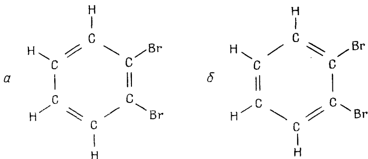
Ф и г. 8.7. Две возможности для орто-дибромбензола.
