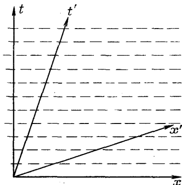
Ф и г. 5.1. Релятивистское преобразование амплитуды покоящейся частицы в систему x-t .
