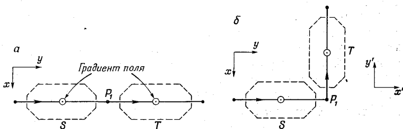
Фиг. 4.4. Поворот на 90^\circ вокруг оси z .
