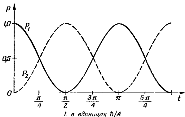
Ф и г. 6.2. P_1 — вероятность того, что молекула аммиака, нагндившаяся при t=0 в состоянии |I\rangle , будет обнаружена в момент t тоже в состоянии |I\rangle ; P_2 — вероятность того, что она будет обнаружена в состоянии |2\rangle .
