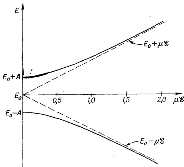
Ф и г. 7.2. Уровни энергии молекул аммиака в электрическом поле.
