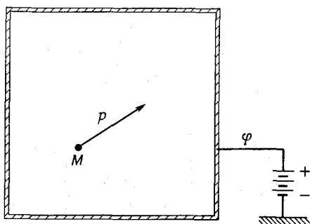
Фиг. 5.2. Частица с массой M и импульсом p в области постоянного потенциала.
