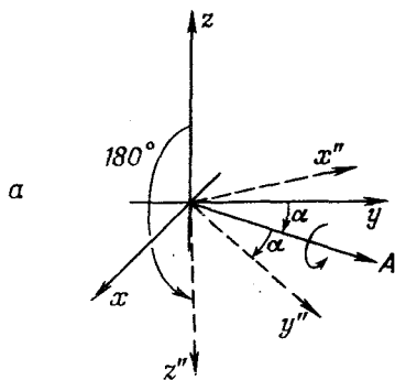
Фиг. 4.7. Поворот на 180^\circ вокруг оси A (а) эквивалентен повороту на 180^\circ вокруг оси y (б), за которым следует поворот вокруг оси z' (в).
