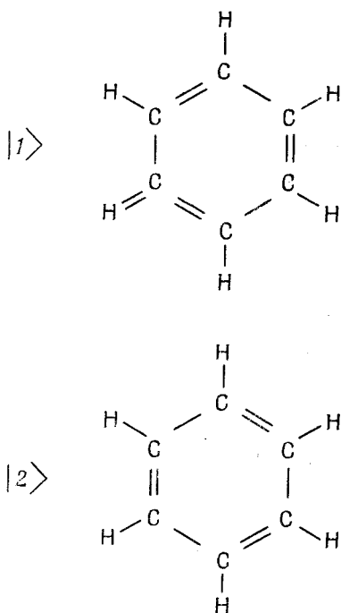
Фиг. 8.8. Совокупность базисных состояний для молекулы бензола.
