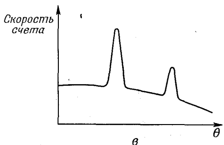
Ф и г. 1.6. Скорость счета нейтронов как функция угла. a — для ядер со спином 0; b — вероятность рассеяния с переворотом спина; v — наблюдаемая скорость счета для ядра со спином 1/2 .
