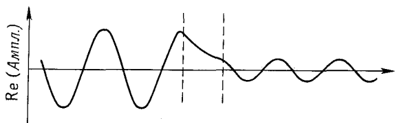
Фиг. 5.5. Проникновение амплитуды сквозь потенциальный барьер.
