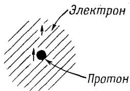
Ф и г. 10.1. Совокупность базисных состояний для основного состояния атома водорода. Эти состояния мы обозначаем |+\rangle , |+\rightarrow\rangle , |-\rangle , |-\rightarrow\rangle .
