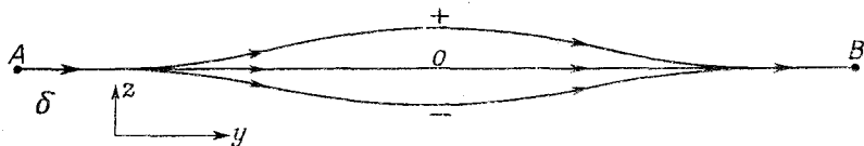
Фиг. 3.3. Воображаемое видоизменение прибора Штерна — Герлаха (а) и пути атомов со спином 1 (б).
