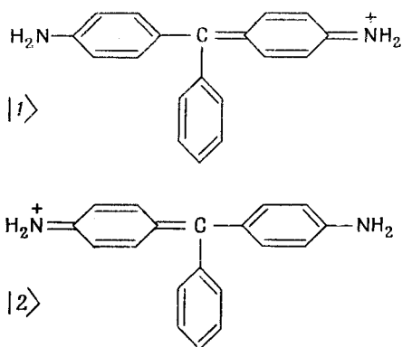
Фиг. 8.9. Пара базисных состояний для молекулы красителя фуксина.
