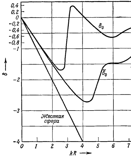
Фиг. 47. Зависимость фазы \delta_0 от kR для случая l=0 при аномальном рассеянии, которое вызвано потенциальной ямой внутри рассеивающей сферы. Для сравнения приведена фаза рассеяния \bar{\delta}_0 , в отсутствие потенциальной ямы, определенная в предыдущей задаче. Прямая линия получена для рассеяния на жесткой сфере.
