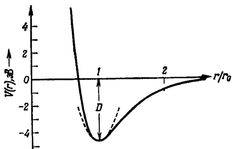
Ф и г. 41. Потенциал Морса для молекулы HCl. Пунктирная кривая — аппроксимирующая параболы.
