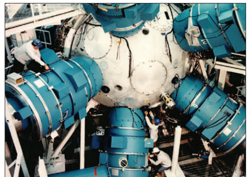
Рис. 2.3. Установка «Шива» для ЛТС
