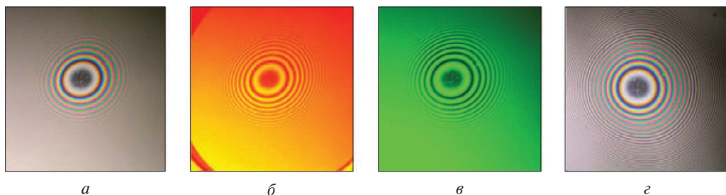
Рис. 9.2. Кольца Ньютона при освещении:
