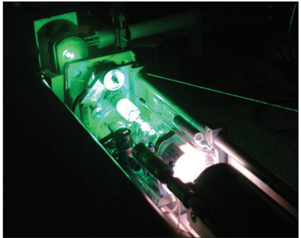
Рис. 7.3. Аргонный лазер
