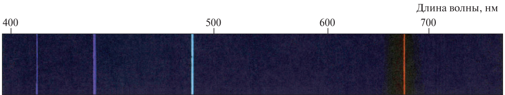
Рис. 5.1. Спектр испускания водорода
