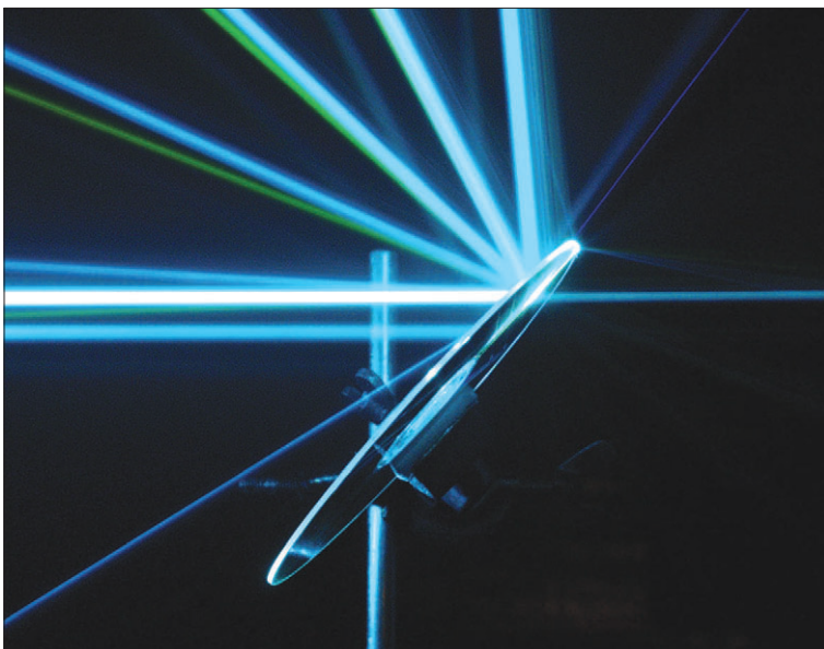
Рис. 13.2. Дифракция пучка аргонового лазера на CD-диске
