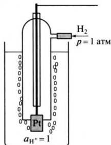
Рис. 7.3. Стандартный водородный электрод
