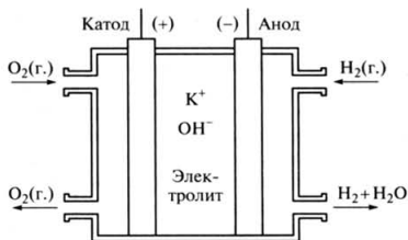
Рис. 7.9. Схема водородно-кислородного топливного элемента
