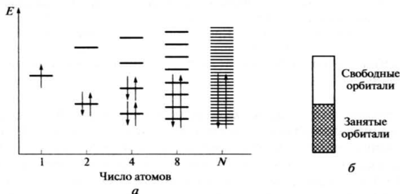
Рис. 9.31. Образование энергетической зоны при увеличении числа химически связанных атомов ( а ); заполнение электронами энергетической зоны вещества с металлическим типом связи ( б )
