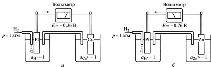
Рис. 7.4. Схема гальванического элемента для измерения стандартного электродного потенциала меди (а) и цинка (б)
