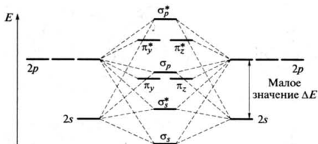
Рис. 9.15. Энергетическая диаграмма молекулярных орбиталей гомоядерных двух-атомных молекул второго периода при малой разности энергий 2s - и 2p -подуровней взаимодействующих атомов
