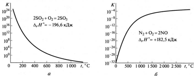
Рис. 4.3. Температурная зависимость константы равновесия экзотермической (а) и эндотермической (б) реакции
