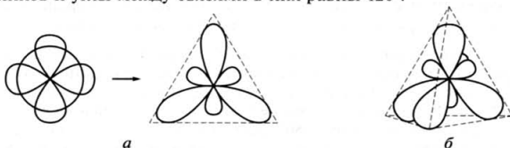
Рис. 9.7. Гибридизация sp^2 -типа ( a ) и sp^3 -типа ( b )
