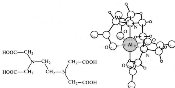
Рис. 11.2. Строение молекулы этилендиаминтетрауксусной кислоты и комплекса иона Al^{3+} с анионом этой кислоты
