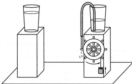
Рис. 2.8. Иллюстрация возможности получения работы при вытекании воды из стакана
