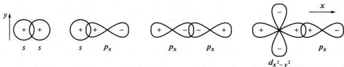
Рис. 9.3. \sigma -Перекрывание атомных орбиталей (за ось x принято направление линии связи)
