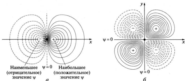
Рис. 8.3. Изолинии 2p_x -орбиталей (а) и 3d_{xy} -орбиталей (б) (в центре системы координат расположено атомное ядро)
