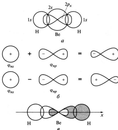
Рис. 9.6. sp -Гибридизация в молекуле \text{BeH}_2 :
