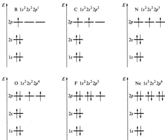
Рис. 8.11. Энергетические диаграммы и электронные конфигурации атомов бора, углерода, азота, кислорода, фтора и неона
