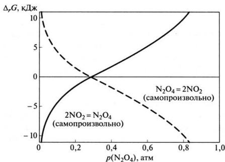
Рис. 4.2. Энергия Гиббса прямой реакции 2\text{NO}_2 \rightarrow \text{N}_2\text{O}_4 (сплошная линия) и обратной реакции \text{N}_2\text{O}_4 \rightarrow 2\text{NO}_2 (пунктирная линия)
