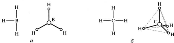
Рис. 9.25. Структурные формулы и геометрическое строение молекул \text{BH}_3 ( а ) и \text{CH}_4 ( б )
