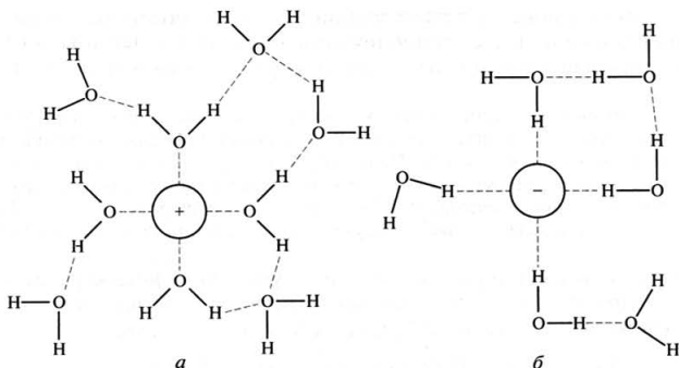
Рис. 5.2. Гидратация катионов (а) и анионов (б) в водных растворах
