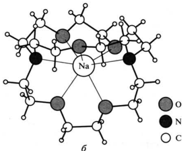
Рис. 11.3. Макроциклический лиганд [2.2.1]-криптант (а) и строение его комплекса с ионом \text{Na}^+ (б)
