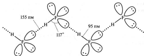
Рис. 10.5. Водородные связи в кристаллическом фтороводороде
