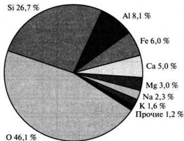
Рис. 12.1. Диаграмма распространенности элементов в земной коре
