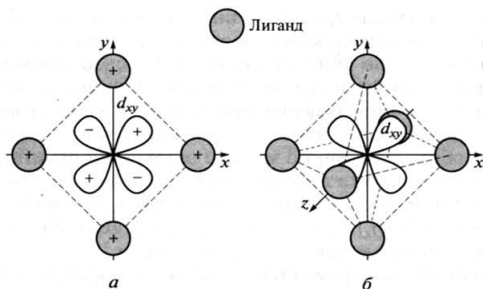
Рис. 11.9. Пример неэффективного \sigma -перекрывания с участием d -орбитали:
