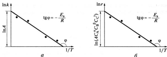
Рис. 3.8. Определение энергии активации E_a и предэкспоненциального множителя A химической реакции графическим методом:
