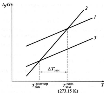
Рис. 5.5. Температурная зависимость энергии Гиббса образования \Delta_f G жидкой воды (1), льда (2), воды в растворе (3)
