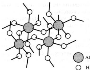
Рис. 14.1. Фрагмент структуры гидрида алюминия (\text{AlH}_3)_n
