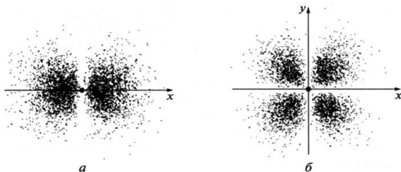
Рис. 8.2. Распределение электронной плотности для 2p_x -орбитали (а) и 3d_{xy} -орбитали (б) в виде сгущения точек (в центре системы координат расположено атомное ядро)
