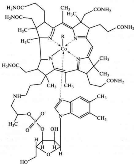
Рис. 28.2. Строение молекулы витамина \text{B}_{12} ( \text{R} = \text{OH}, \text{CH}_3 )
