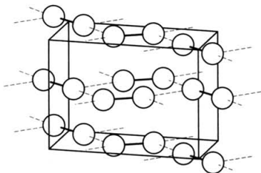
Рис. 10.4. Упаковка молекул I_2 в элементарной ячейке кристаллического иода (пунктиром показаны кратчайшие межмолекулярные контакты)
