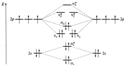
Рис. 18.1. Энергетическая диаграмма молекулярных орбиталей молекулы \text{N}_2
