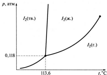
Рис. 4.6. Диаграмма состояния иода (схема)
