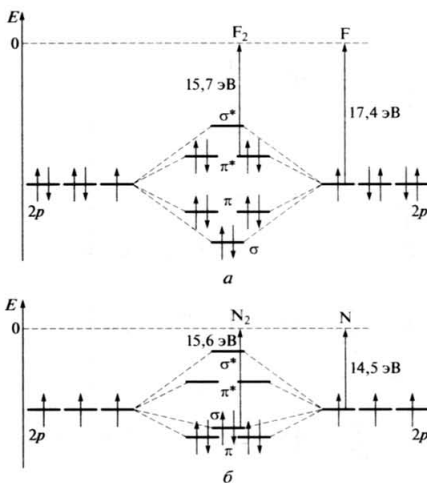
Рис. 9.17. Сравнение энергий ионизации молекул F_2 (а) и N_2 (б) с энергиями ионизации атомов F и N
