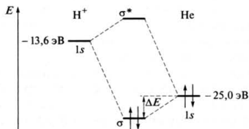
Рис. 9.13. Энергетическая диаграмма молекулярных орбиталей иона \text{HeH}^+
