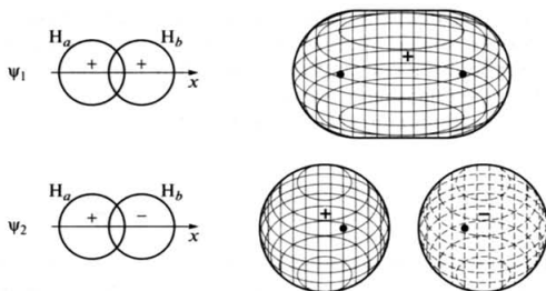
Рис. 9.10. Граничные поверхности молекулярных орбиталей в молекуле водорода H_2 (точками показано положение атомных ядер)
