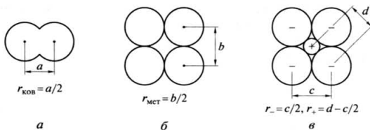
Рис. 9.30. Способы определения ковалентных (а), металлических (б) и ионных (в) радиусов
