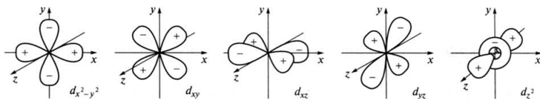
Рис. 8.8. Схематическое изображение граничных поверхностей d -орбиталей
