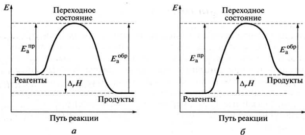
Рис. 4.4. Энергетический профиль экзотермической (а) и эндотермической (б) реакции
