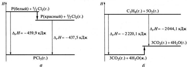
Рис. 2.4. Энтальпийные диаграммы реакций:
