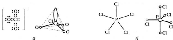
Рис. 9.28. Положение электронных пар и геометрическое строение иона \text{ClO}_3^- (а) и молекулы \text{PCl}_5 (б)
