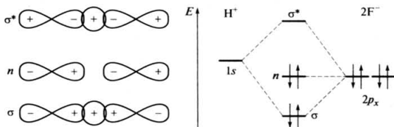
Рис. 9.22. Схема образования молекулярных орбиталей и фрагмент энергетической диаграммы молекулярных орбиталей аниона HF 2 - (показаны только атомные орбитали, участвующие в связывании)
