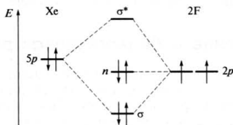
Рис. 32.2. Энергетическая диаграмма молекулярных орбиталей молекулы XeF_2
