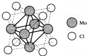
Рис. 26.1. Строение иона [\text{Mo}_6\text{Cl}_8]^{4+} в составе дихлорида молибдена
