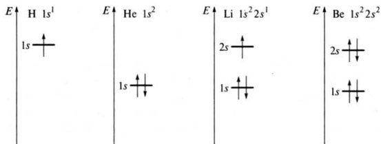
Рис. 8.10. Энергетические диаграммы и электронные конфигурации атомов водорода, гелия, лития и бериллия
