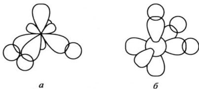
Рис. 9.8. Образование химических связей:
