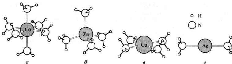
Рис. 11.1. Строение комплексных частиц:
