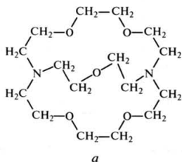
Рис. 11.3. Макроциклический лиганд [2.2.1]-криптант (а) и строение его комплекса с ионом \text{Na}^+ (б)
