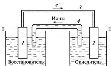
Рис. 7.1. Схема гальванического элемента:
