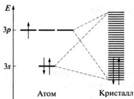
Рис. 9.32. Образование энергетической зоны в кристаллах алюминия
