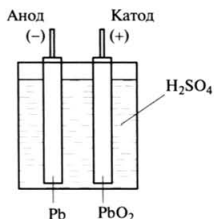
Рис. 7.8. Схема свинцового аккумулятора
