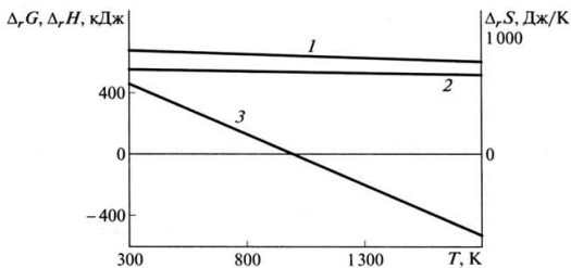
Рис. 2.9. Температурные зависимости энтальпии \Delta_r H (1), энтропии \Delta_r S (2) и энергии Гиббса \Delta_r G (3) реакции \text{Fe}_3\text{O}_4 + 4\text{C} = 3\text{Fe} + 4\text{CO}
