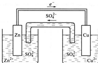
Рис. 7.6. Схема элемента Даниэля
