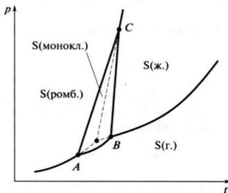
Рис. 17.1. Схема фазовой диаграммы серы: S(ромб.) — ромбическая кристаллическая модификация, S(монокл.) — моноклинная. Тройные точки: A ( t = 95,5^\circ\text{C} , p = 4,9 \cdot 10^{-6} атм); B ( t = 119,3^\circ\text{C} , p = 3,3 \cdot 10^{-5} атм); C ( t = 151^\circ\text{C} , p = 1288 атм)
