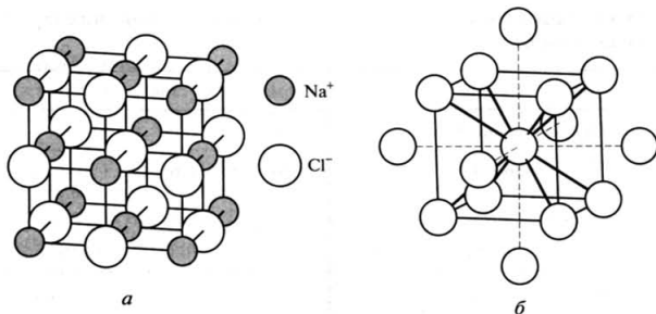
Рис. 9.29. Модели кристаллических структур хлорида натрия ( a ) и \alpha -железа ( б )
