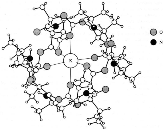
Рис. 11.4. Строение комплекса катиона \text{K}^+ с молекулой валиномицина
