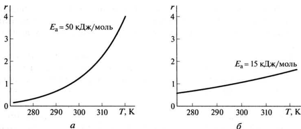
Рис. 3.5. Изменение скорости химической реакции в зависимости от температуры при большой (а) и малой (б) энергии активации (скорость реакции при T = 298\text{ K} принята за единицу)
