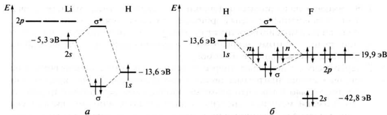
Рис. 9.19. Энергетические диаграммы молекулярных орбиталей молекул LiH (а) и HF (б)
