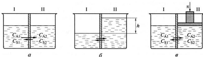
Рис. 5.6. Иллюстрация явления осмоса:
