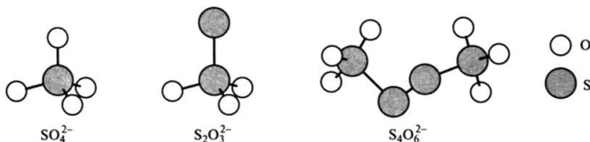
Рис. 17.3. Строение анионов \text{SO}_4^{2-} , \text{S}_2\text{O}_3^{2-} , \text{S}_4\text{O}_6^{2-}
