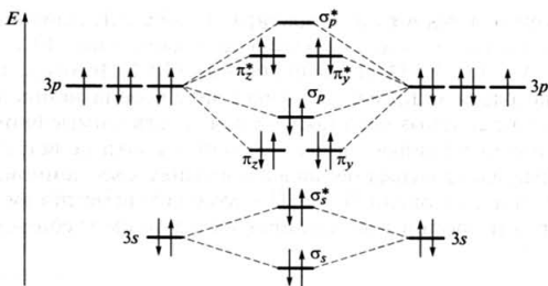
Рис. 16.1. Энергетическая диаграмма молекулярных орбиталей молекулы \text{Cl}_2
