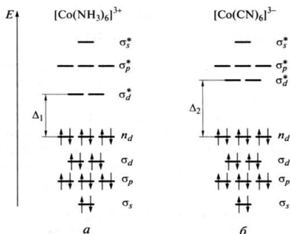
Рис. 11.12. Энергетические диаграммы молекулярных орбиталей комплексов [\text{Co}(\text{NH}_3)_6]^{3+} (а) и [\text{Co}(\text{CN})_6]^{3-} (б)
