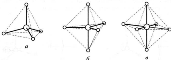
Рис. 9.23. Многогранники:
