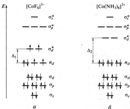
Рис. 11.11. Распределение электронов по молекулярным орбиталям в комплексах с лигандами слабого поля [\text{CoF}_6]^{3-} (а) и сильного поля [\text{Co}(\text{NH}_3)_6]^{3+} (б)
