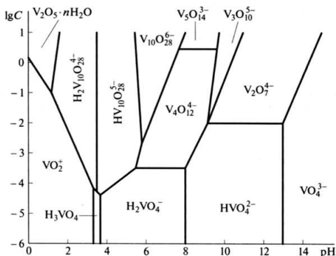
Рис. 25.2. Формы существования ванадия(V) в зависимости от его концентрации и pH среды
