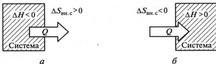
Рис. 2.7. Изменение энтальпии системы \Delta H и энтропии внешней среды \Delta S_{\text{вн.с}} в экзотермических (а) и эндотермических (б) реакциях
