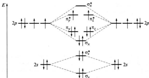
Рис. 15.1. Энергетическая диаграмма молекулярных орбиталей молекулы O_2
