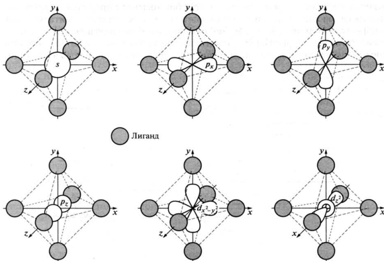
Рис. 11.8. Перекрывание орбиталей комплексообразователя и лигандов в октаэдрическом комплексе, приводящее к образованию координационных связей
