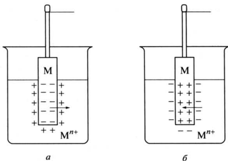
Рис. 7.2. Возникновение электродного потенциала:
