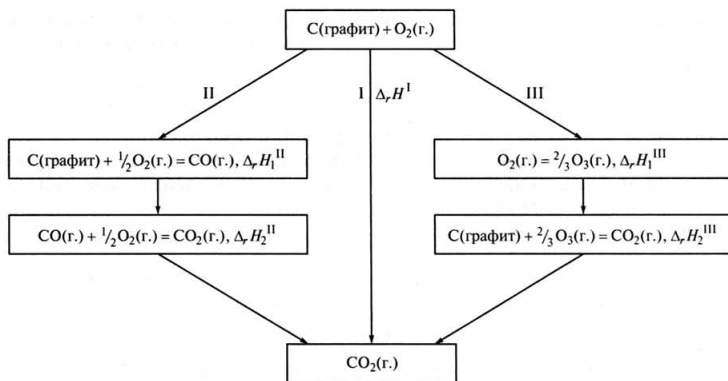
Рис. 2.1. Возможные пути (I—III) получения диоксида углерода
