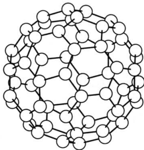
Рис. 22.2. Строение молекулы фуллерена \text{C}_{60}
