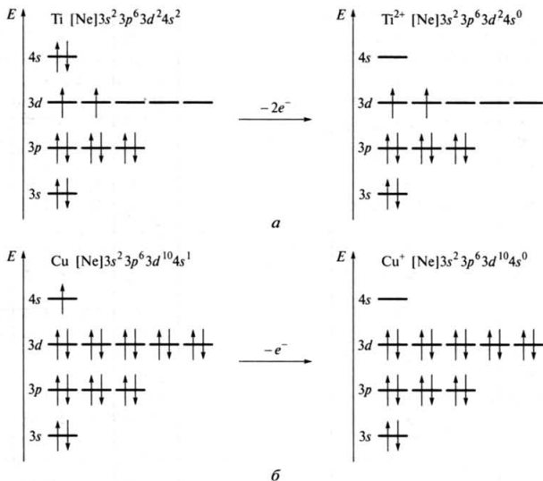
Рис. 8.14. Энергетические диаграммы и электронные конфигурации: а — атом титана и ион \text{Ti}^{2+} ; б — атом меди и ион \text{Cu}^+
