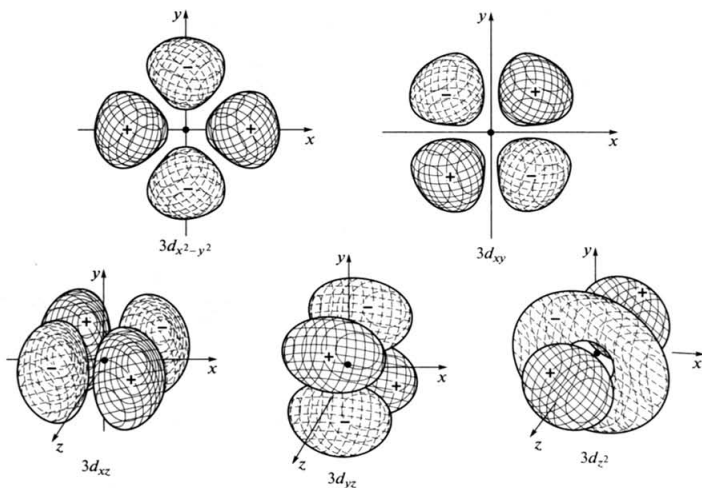
Рис. 8.5. Граничные поверхности 3d -орбиталей (в центре системы координат расположено атомное ядро)
