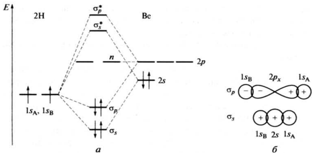
Рис. 9.20. Энергетическая диаграмма молекулы BeH 2 (а) и схемы перекрывания атомных орбиталей (б)
