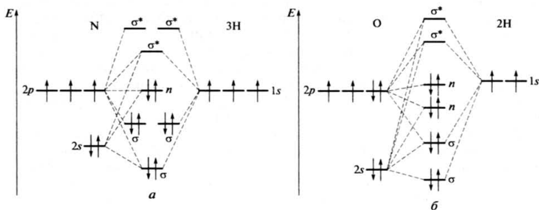
Рис. 9.21. Энергетические диаграммы молекулярных орбиталей молекул NH 3 (а) и H 2 O (б)
