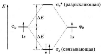
Рис. 9.11. Энергетическая диаграмма молекулярных орбиталей молекулы H_2
