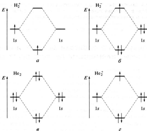
Рис. 9.12. Энергетические диаграммы молекулярных орбиталей:
