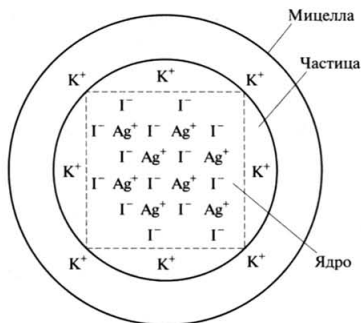
Рис. 6.2. Строение мицеллы золя AgI
