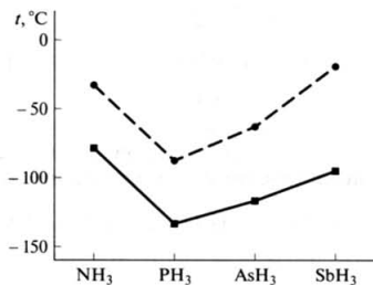
Рис. 18.3. Температуры плавления (сплошная линия) и кипения (пунктирная линия) водородных соединений элементов 15-й группы
