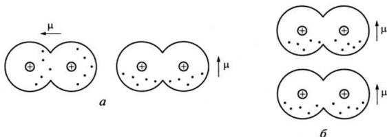
Рис. 10.3. Возникновение «мгновенного» дипольного момента \mu ( а ) у двухатомной неполярной молекулы (положение электронов обозначено точками); взаимное притяжение «мгновенных» диполей ( б ) при согласованном движении электронов
