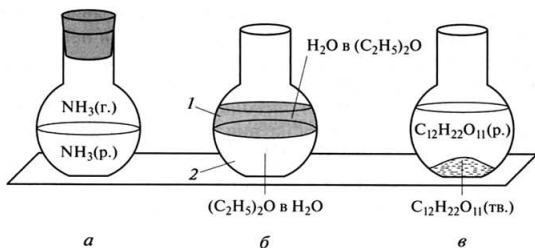
Рис. 5.1. Равновесия в насыщенных растворах:
