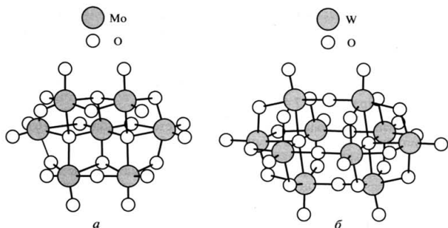
Рис. 26.2. Структура изополианионов [\text{Mo}_7\text{O}_{24}]^{6-} (а) и [\text{W}_{10}\text{O}_{32}]^{4-} (б)
