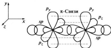
Рис. 9.9. Образование \sigma - и \pi -связей в молекуле ацетилена \text{H}-\text{C}\equiv\text{C}-\text{H}
