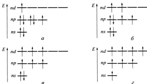
Рис. 32.1. Расположение валентных электронов на атомных орбиталях благородных газов при образовании ими двух (а), четырех (б), шести (в) и восьми (г) химических связей
