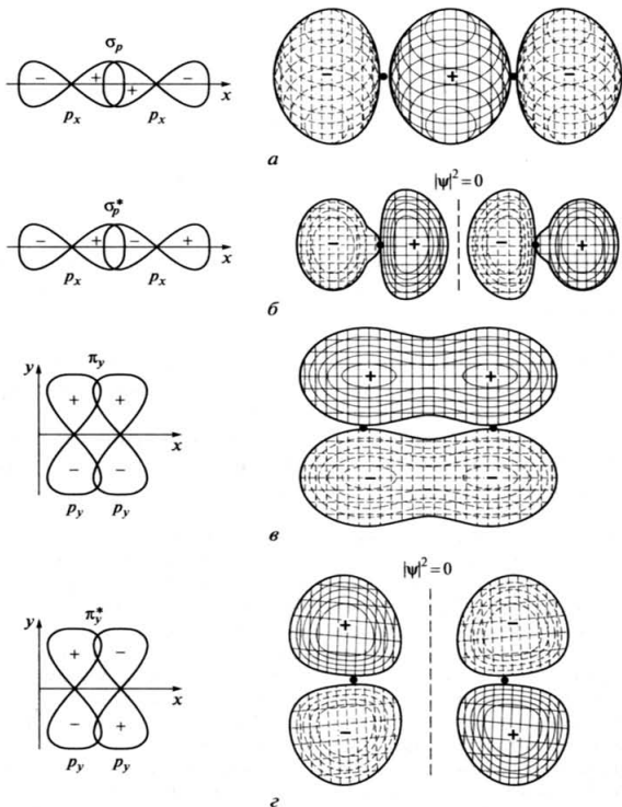
Рис. 9.14. Граничные поверхности связывающих и разрыхляющих молекулярных \sigma - и \pi -орбиталей, образующихся при перекрывании атомных 2p -орбиталей:
