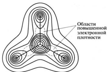
Рис. 9.24. Распределение электронной плотности в молекуле \text{BH}_3
