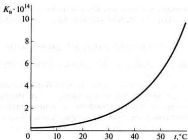
Рис. 6.1. Зависимость ионного произведения воды K_b от температуры
