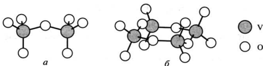
Рис. 25.1. Строение ванадат-ионов V_2O_7^{4-} (а), V_4O_{12}^{4-} (б)
