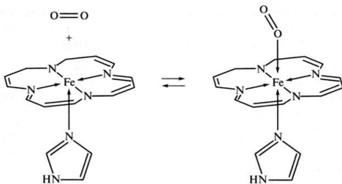
Рис. 28.1. Комплекс железа с гемоглобином, взаимодействующий с молекулой кислорода
