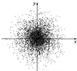
Рис. 8.1. Распределение электронной плотности для 1s -орбитали атома водорода
