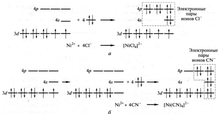
Рис. 11.6. Распределение электронов по атомным орбиталим иона \text{Ni}^{2+} :
