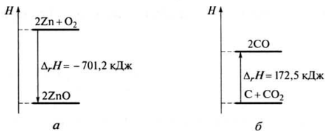
Рис. 2.3. Изменение энтальпии системы:
