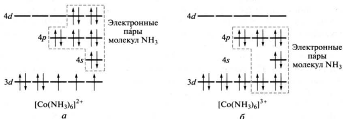
Рис. 11.7. Распределение электронов по атомным орбиталим комплексообразователя: а — в комплексе [\text{Co}(\text{NH}_3)_6]^{2+} ; б — в комплексе [\text{Co}(\text{NH}_3)_6]^{3+}
