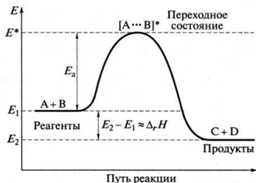
Рис. 3.6. Энергетический профиль элементарной химической реакции A + B = C + D
