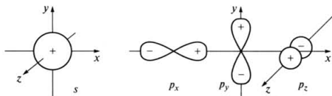
Рис. 8.7. Схематическое изображение граничных поверхностей s - и p -орбиталей
