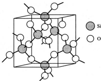
Рис. 22.3. Кристаллическая структура кварца
