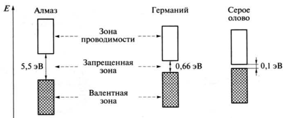
Рис. 9.33. Энергетические зоны в кристаллах диэлектрика — алмаза и полупроводников — германия и серого олова
