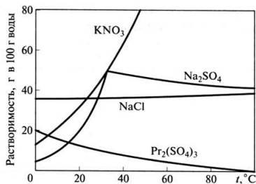
Рис. 5.3. Зависимость растворимости некоторых солей (в граммах растворенного вещества в 100 г воды) от температуры
