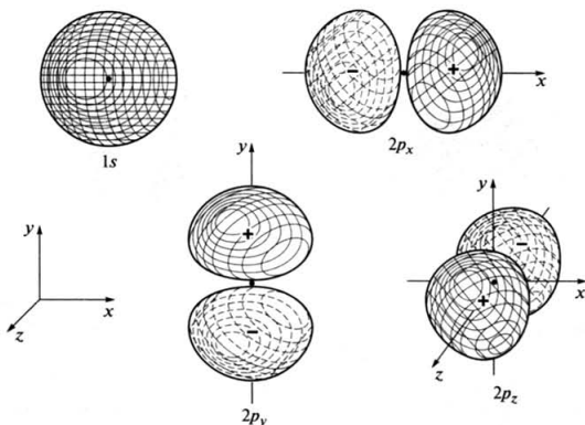
Рис. 8.4. Граничные поверхности 1s -, 2p_x -, 2p_y - и 2p_z -орбиталей (в центре системы координат расположено атомное ядро)
