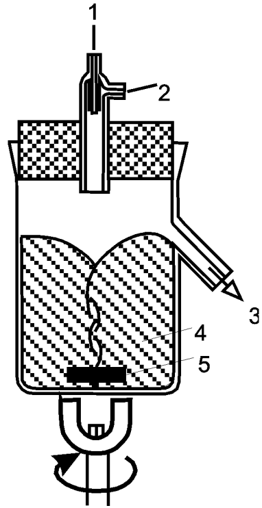
Рис. 11.2. 1 — регулятор, 2 — поступление субстрата, 3 — отток (вымывание) смеси субстрата и биомассы, 4 — культура внутри культиватора, 5 — мешалка.
