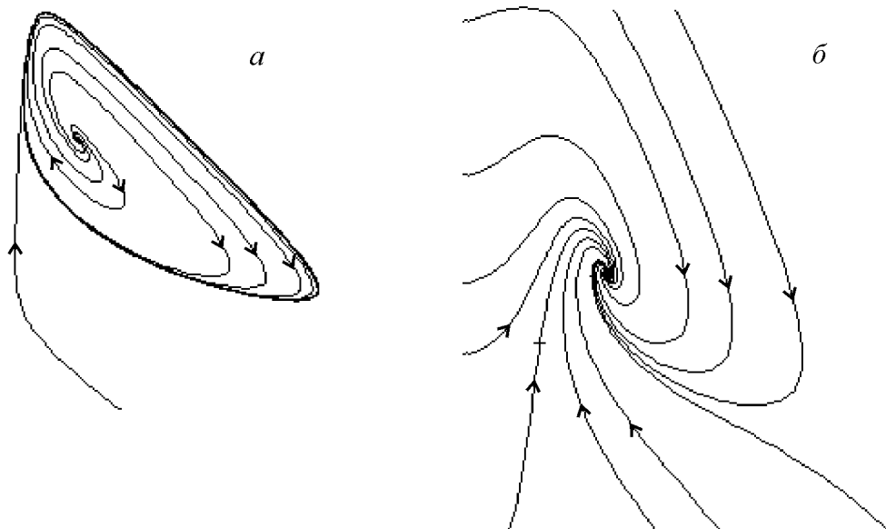
Рис. 8.9. Фазовый портрет системы брусслетор при B > 1 + A^2 (а) и B < 1 + A^2 (б).
