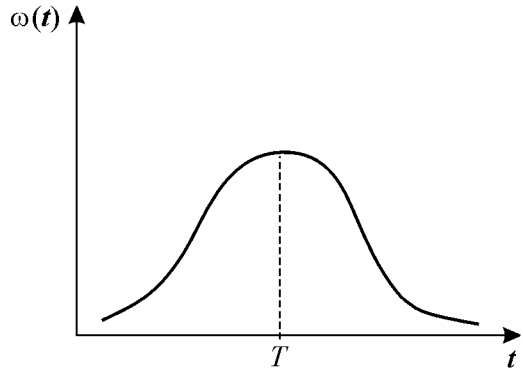
Рис. 3.20. Весовая функция распределения времени запаздывания для уравнения 3.25.
