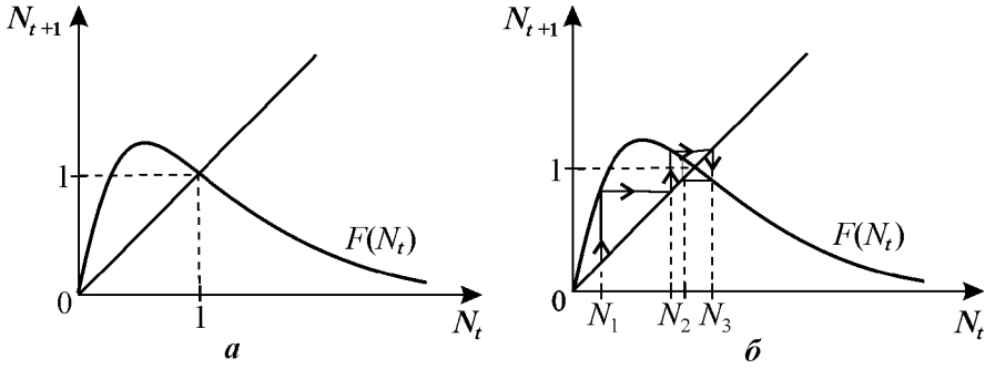
Рис. 3.12. Определение равновесного состояния в дискретной модели популяции с непрерывными поколениями — диаграмма (а) и лестница Ламерея (б)
