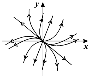
Неустойчивый узел. ( \lambda_1, \lambda_2 действительны и положительные)
