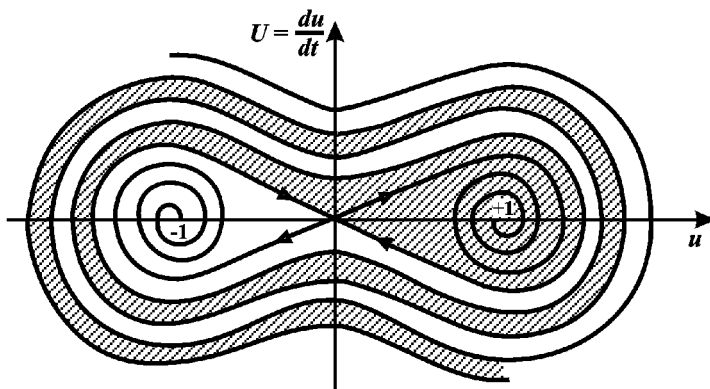
Рис. 7.2. Фазовый портрет системы 7.2 (шарик в ложбине с двумя лунками). Темным обозначена область притяжения стационарного состояния (+1) (Д. С. Чернавский, 1986).
