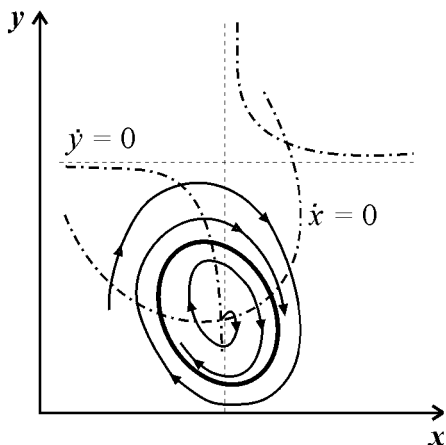
Рис. 9.7. Фазовый портрет модели (9.16) (MacArthur, 1971). Жирная замкнутая кривая — предельный цикл, штрих-пунктир — изоклины вертикальных и горизонтальных касательных.
