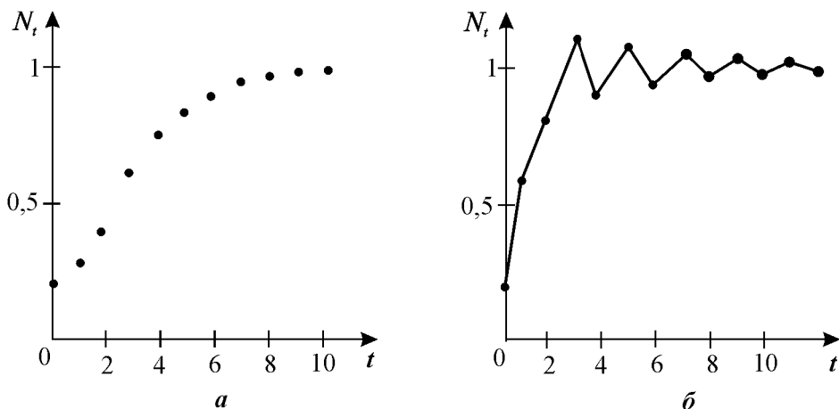
Рис. 3.13. Графики численности популяции, вычисленные по формуле (3.13) при выполнении условия (3.14). Устойчивое состояние равновесия; a — монотонный рост, b — затухающие колебания.
