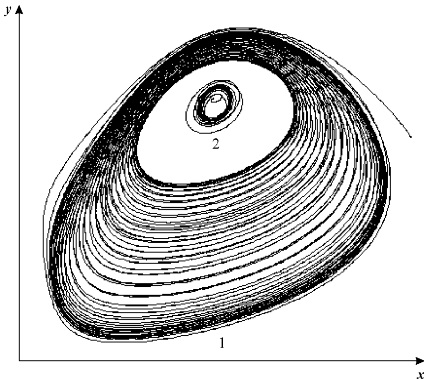
Рис. 12.10. Квазихаотический режим. V_K = 0,5 , k_H = 0,01 , b = 1 , c = 1 , V_H = 0,7065 , A = 0,003 , \omega = 0,0025 .
