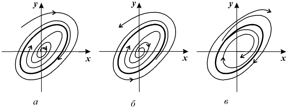
Рис. 8.2. Устойчивый (а) и неустойчивые (б и в) предельные циклы на фазовой плоскости.
