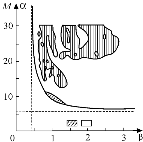
Рис. 10.11. Области стохастичности (штриховка) для системы (10.19): два хищника — две жертвы. (Алексеев, Лоскутов, 1985.)
