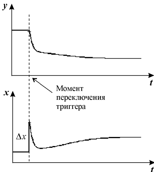
Рис. 7.4. Поведение переменных во времени при силовом переключении после добавления в систему вещества x в количестве, достаточном для переключения системы из режима a в режим c (смотри рис. 7.3).
