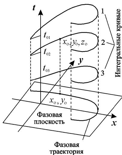
Рис. 4.3. Траектории системы в пространстве (x, y, t) .
