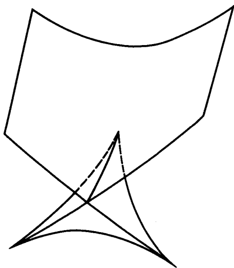
Рис. 6.9. Бифуркация «ласточкин хвост».
