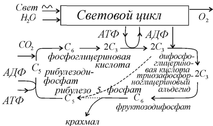
Рис. 8.11. Упрощенная схема цикла Кальвина темновых реакций фотосинтеза — превращения углекислоты в углеводы.
