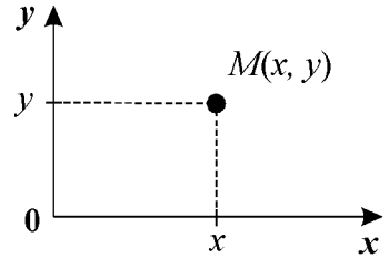
Рис. 4.1. Изображающая точка на фазовой плоскости.
