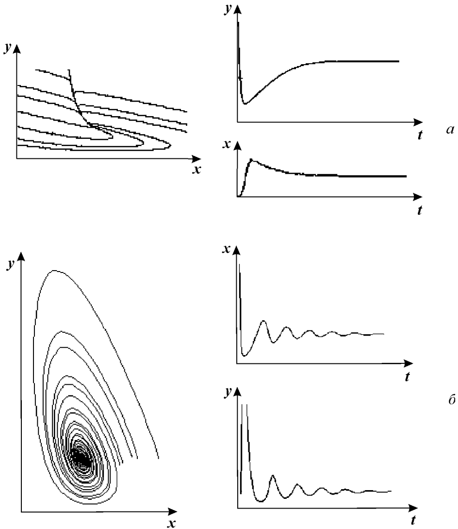
Рис. 8.14 a, б . Модель гликолиза (8.10). Кинетика изменений концентраций фруктозо-6-фосфата ( x ) и фруктозодифосфата ( y ) (справа) и фазовый портрет системы (слева) при разных значениях параметров системы, a — бесколебательный процесс (узел на фазовой плоскости), \alpha = 0,25 ; r = 1 . б — затухающие колебания (устойчивый фокус на фазовой плоскости) \alpha = 4 ; r = 0,2 .
