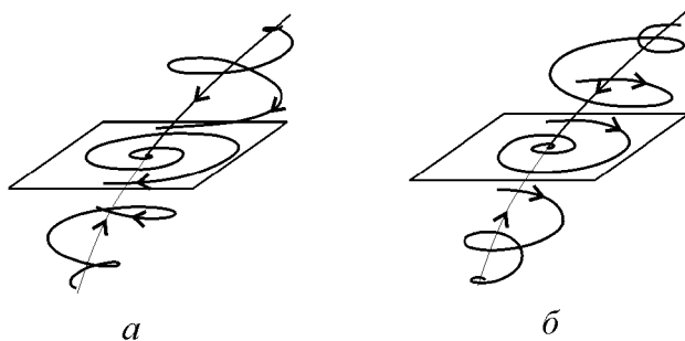
Рис. 10.2. Седло-фокусы в пространстве N = 3 . а) p_1 — действительно и отрицательно, p_{2,3} — комплексно сопряженные, \text{Re } p_{2,3} > 0 ; б) p_1 — действительно и положительно, p_{2,3} — комплексно сопряженные, \text{Re } p_{2,3} < 0 .
