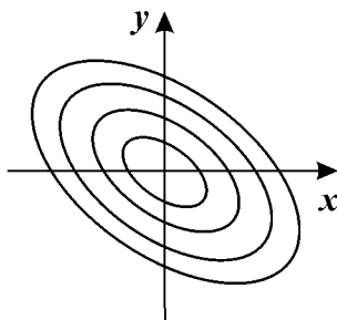
Центр. ( \lambda_1, \lambda_2 - чисто мнимые)
