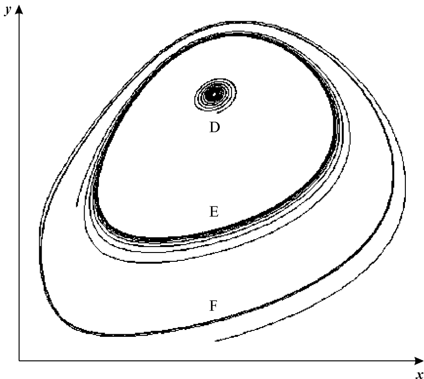
Рис. 12.9. Фазовый портрет невозмущенной системы вблизи большого критического значения параметра V_H . В интервале значений V_H = 0,701-0,7065 в системе одновременно существуют устойчивый фокус D , неустойчивый предельный цикл E , устойчивый предельный цикл F . V_K = 0,5 , k_H = 0,01 , b = 1 , c = 1 .
