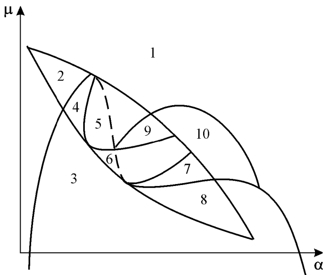
Рис. 9.8. Параметрический портрет системы (9.18) при фиксированных \gamma и малых \varepsilon .
