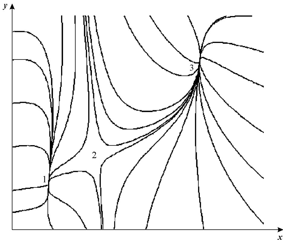
Рис. 12.5. Фазовый портрет системы (12.10). V_H = 10,637 , V_K = 0,0325 , k_H = 1 , a = 26,44 , b = 0,696 .
