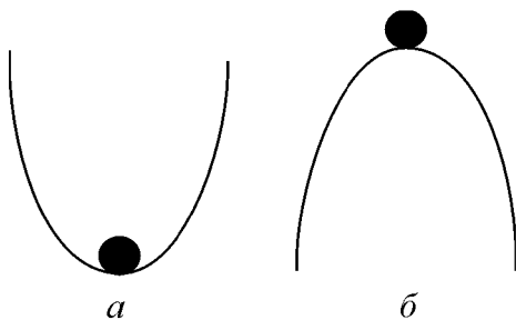
Рис. 2.3. К понятию устойчивости состояния равновесия.
