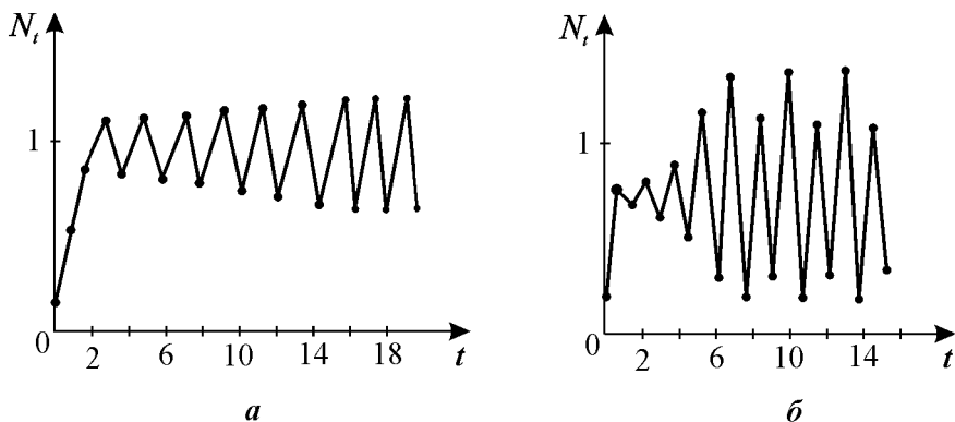
Рис. 3.14. Циклическое поведение решения уравнения 3.13, a — двухточечный цикл, b — четырехточечный цикл.
