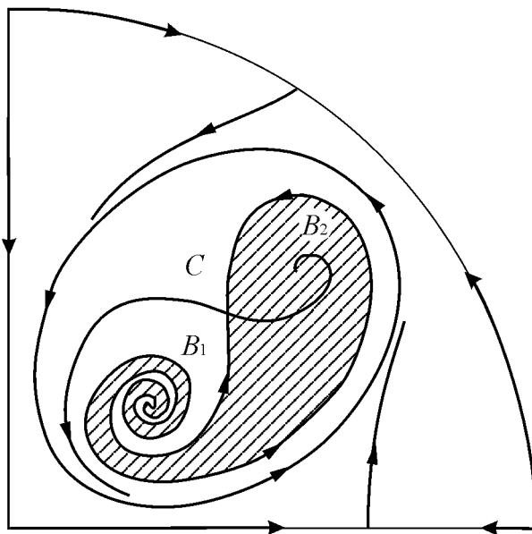
Рис. 9.10. Фазовый портрет системы 9.18 для параметрической области \delta . Область притяжения B_2 заштрихована.
