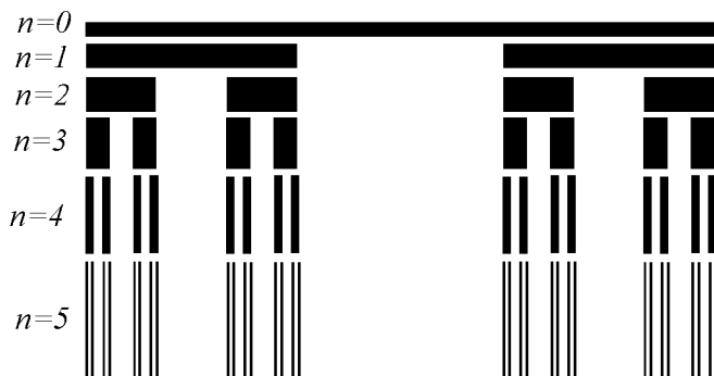
Рис. П.5. Триадный канторовский стержень. Высота стержня в n -м поколении пропорциональна его плотности.
