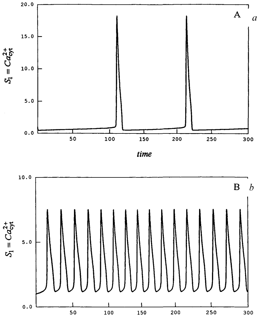
Рис. 8.16. Модель внутриклеточных колебаний кальция. Кинетика концентрации Ca при разных значениях параметров. a — k_5 = 1 , v_0 = 1,4 , b — k_5 = 1 , v_0 = 3,0 . (Dupont, Goldbeter, 1983.)
