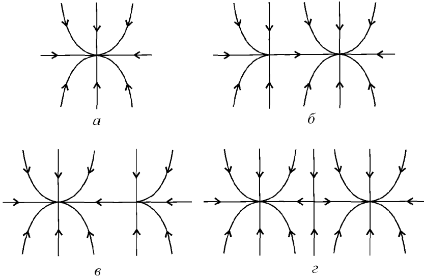
Рис. 6.7. Трансформации фазового портрета при бифуркации «рождение двух узлов из седла». a — фазовый портрет в незаштрихованной области (рис. 6.8 a ); б — фазовый портрет на границе l_1 ; в — фазовый портрет на границе l_2 ; г — фазовый портрет в заштрихованной области представлен двумя устойчивыми узлами и седлом между ними.
