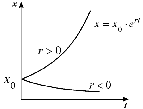
Рис. 2.5. Экспоненциальная форма динамики роста численности колонии микроорганизмов в соответствии с системой уравнений (2.7).
