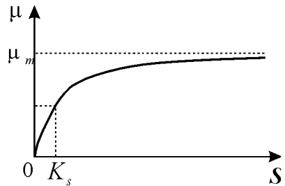
Рис. 11.3. График зависимости скорости роста от концентрации субстрата в соответствии с формулой Моно (11.4).
