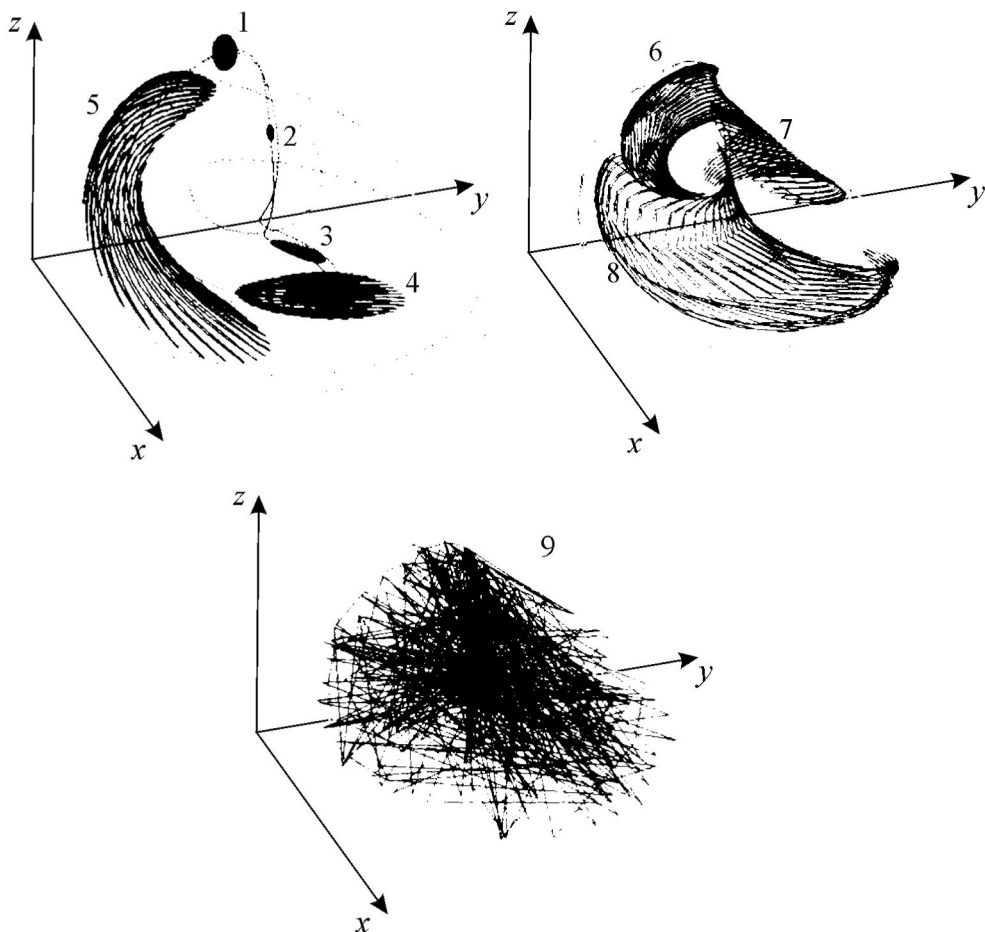
Рис. 10.8. Перемешивание в квазистохастической системе. Эволюция малого первоначального фазового объема во времени в динамической системе (10.12). (Анищенко и др., 1999.)
