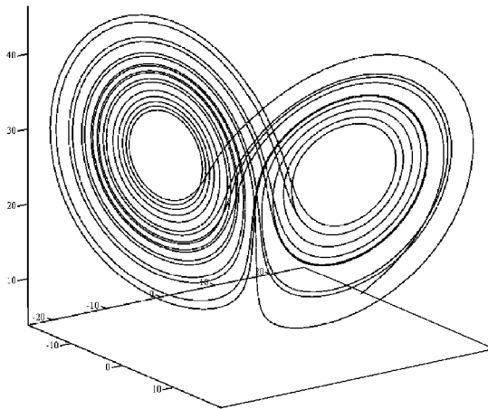
Рис. 10.1. Хаотические траектории в системе Лоренца.
