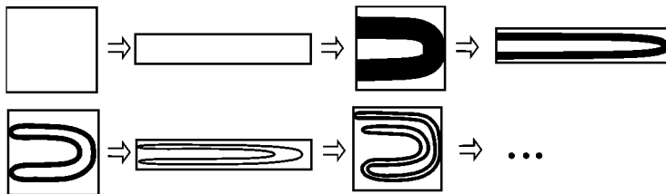
Рис. 10.5. Возникновение странного аттрактора в отображении подковы (Смейла).
