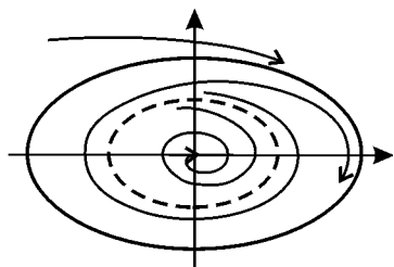
Рис. 8.5. Фазовый портрет системы, имеющий устойчивый и неустойчивый (пунктир) предельные циклы.
