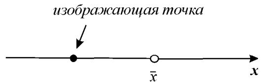
Рис. 2.2. Фазовая прямая.
