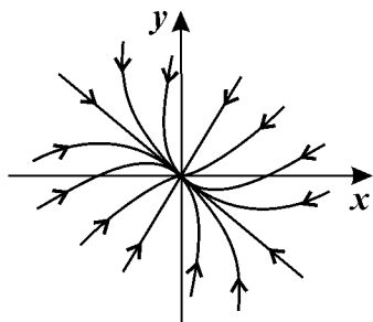
Устойчивый узел. ( \lambda_1, \lambda_2 действительны и отрицательны)
