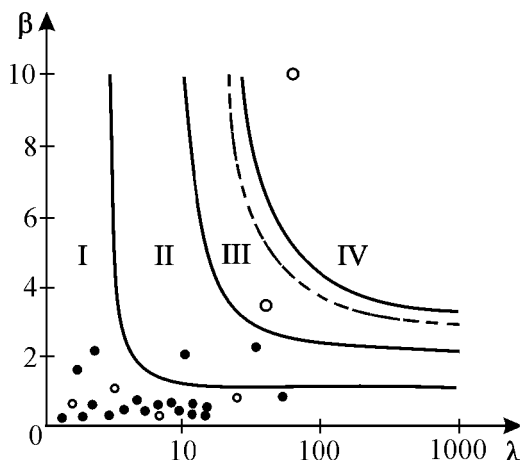
Рис. 3.17. Области значений параметров для уравнения 3.17 с различным характером поведения. Точками указаны значения параметров для реальных популяций (Hassel, 1976).
