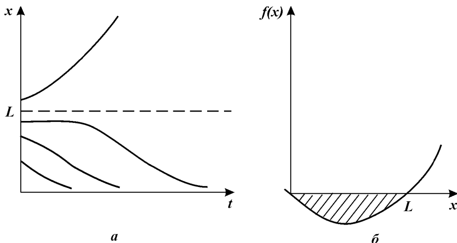
Рис. 3.8. Зависимость численности популяции от времени (а) и скорости роста от численности (б) для уравнения (3.8). Штриховкой обозначена область вырождения популяции.
