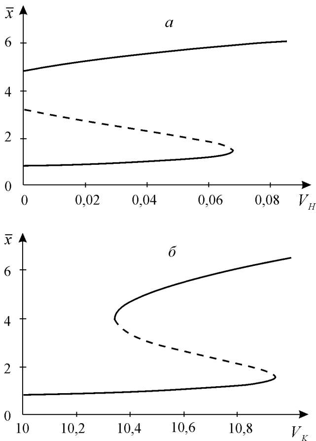
Рис. 12.4. Зависимость стационарной концентрации протонов \bar{x} от скорости притока протонов V_H (а) и ионов калия V_K (б) в сферу реакции.
