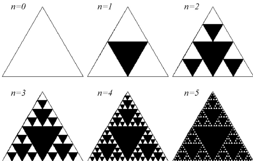
Рис. П.2. Построение треугольной салфетки Серпинского. Начальный элемент — треугольник со всеми внутренними точками. Образующий элемент исключает из него центральный треугольник. На рисунке показаны пять поколений предфракталов. Фрактальное множество получается в пределе при бесконечно большом числе поколений и имеет фрактальную размерность D = \ln 3 / \ln 2 = 1,58 \dots
