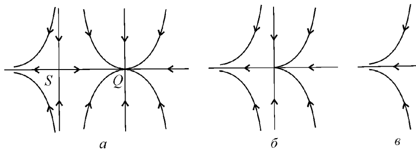
Рис. 6.5. Бифуркация седло–узел.
