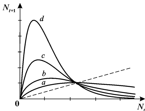
Рис. 3.10. Вид одноэкстремальной функции N_{t+1} = f(N_t) .
