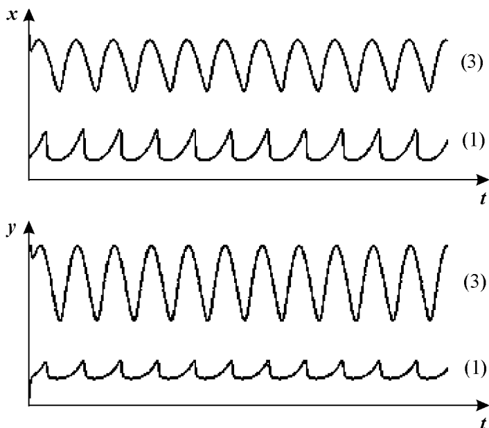
Рис. 12.6 а. Кинетика изменения переменных в бистабильной системе (12.8) при наложении внешнего периодического воздействия. Для кривых (1) начальные значения переменных соответствуют стационарному состоянию 1 (рис. 12.5); для кривых (3) — стационарному состоянию 3 (рис. 12.5). Параметры системы V_H = 10,637 , V_K = 0,0325 , k_H = 1 , a = 26,44 , b = 0,696 , амплитуда внешнего воздействия A = 0,03 , частота воздействия \omega < \omega_1 .
