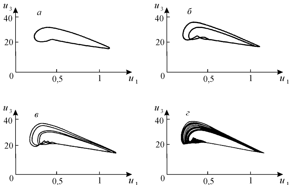
Рис. 10.9. Система (10.15), описывающая взаимодействие трех видов: хищник – две жертвы (А. Д. Базыкин, 1985). При уменьшении параметра скорости роста первой жертвы происходит усложнение траектории (последовательное удвоение предельного цикла) a–г . Колебательная динамика переходит в квазистохастическую.
