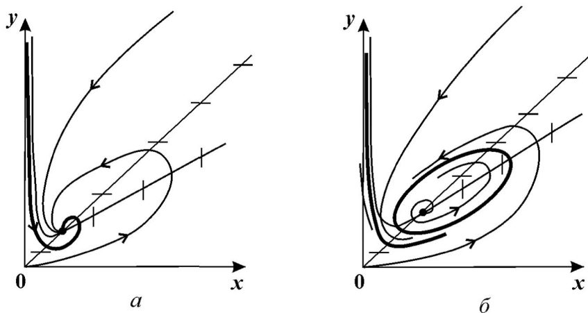
Рис. 8.12. Фазовый портрет системы (8.9) при разных соотношениях параметров (указаны в тексте). a — стационарное состояние (1,1) — устойчивый фокус. b — (1,1) — неустойчивый фокус, жирная кривая — предельный цикл. (Чернавский Н. М., Чернавский Д. С., 1867.)
