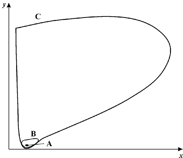
Рис. 12.7. Фазовый портрет системы (12.12) в отсутствие внешнего поля ( A = 0 ) при разных значениях параметра V_H вблизи значений, соответствующих бифуркации Андронова – Хопфа. x, y – безразмерные концентрации протонов и ионов калия, V_K = 0,5, k_H = 0,01, b = 1, c = 1 . При V_H = 0,5241 в системе реализуется устойчивый фокус А, при V_H = 0,5242 возникает предельный цикл В, при V_H = 0,5245 амплитуда цикла резко возрастает, кривая С.
