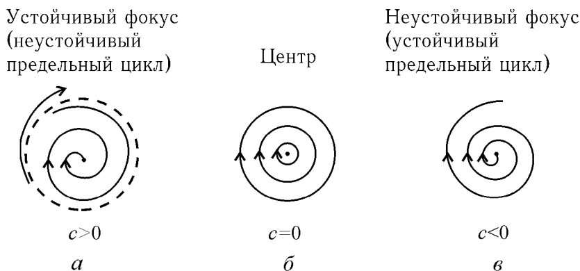
Рис. 8.7. Докритическая (субкритическая) бифуркация Андронова–Хопфа. Жесткое возбуждение автоколебаний. «Локальные события» при изменении параметра при переходе через бифуркационное значение: устойчивый фокус и неустойчивый предельный цикл пунктир (а), при уменьшении параметра c переходят в центр (б), а затем в неустойчивый фокус (в). Внешний большой устойчивый предельный цикл находится за пределами локальной системы, в которой происходит бифуркация.
