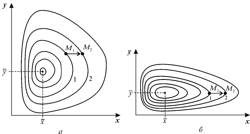
Рис. 5.3. Фазовый портрет системы 5.17. Особая точка типа «центр». a — параметры системы: \varepsilon_x = 4 , \gamma_{xy} = 0,3 , \varepsilon_y = \gamma_{yx} = 0,4 ; b — параметры системы: \varepsilon_x = 2 , \gamma_{xy} = 0,3 , \varepsilon_y = \gamma_{yx} = 0,4 .
