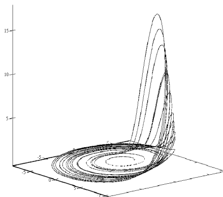
Рис. 10.3. Вид проекций фазовой траектории на странном аттракторе в системе Ресслера.
