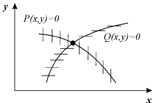
Рис. 4.2. Пересечение главных изоклин на фазовой плоскости.
