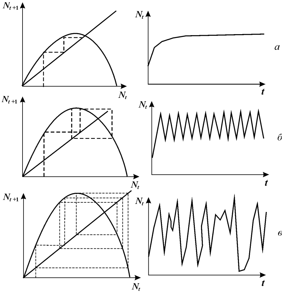
Рис. 3.16. Диаграммы Ламерея и динамика численности во времени для разных значений параметра a в уравнении 3.16. a — монотонный рост; b — двухточечный цикл; b — квазистогастическое поведение.
