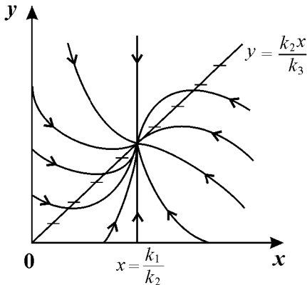
Рис. 4.11. Фазовый портрет системы линейных химических реакций (4.15).
