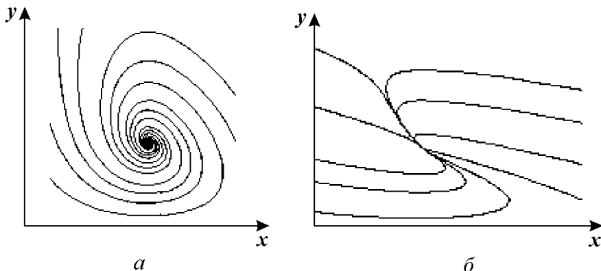
Рис. 5.1. Фазовый портрет системы 5.13. a — устойчивый фокус, k_0 = 2 , k_1 = 10 , k_2 = 2 . б — устойчивый узел. k_0 = 2 , k_1 = 2 , k_2 = 4 .
