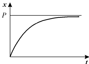
Рис. 2.6. Концентрация вещества x в зависимости от времени. График уравнения 2.9.
