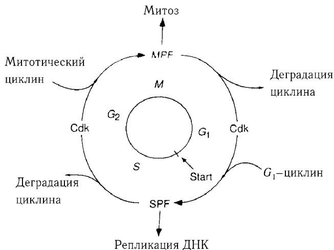
Рис. 8.17. Схема регуляции клеточного цикла.
