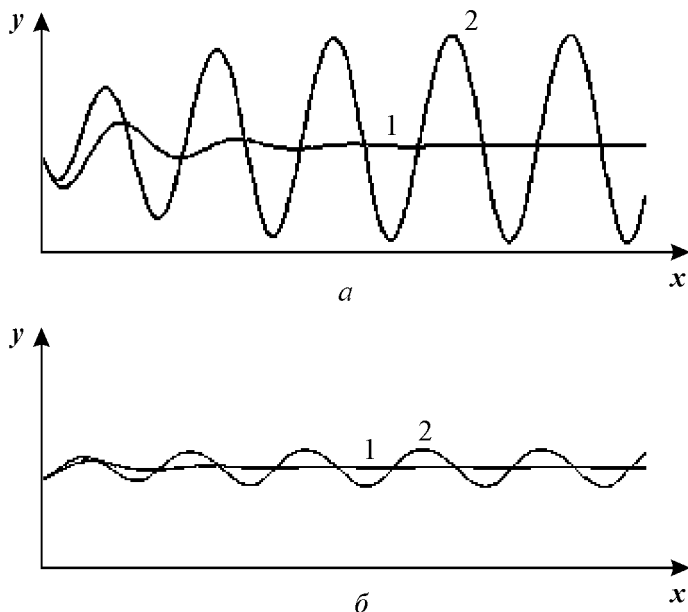
Рис. 12.3. Изменения безразмерных концентраций (а) протонов ( x ) и (б) ионов K^+ ( y ) во времени. Кривые 1 — в соответствии с системой уравнений (12.4), кривые 2 — в соответствии с системой уравнений (12.7) при периодическом воздействии. V_H = 1 , V_K = 0,96 , a = 30 , A = 0,0005 , \omega = 0,064 .
