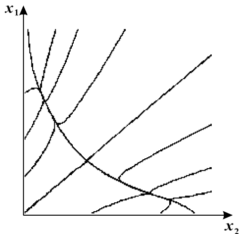
Рис. 7.11. Фазовый портрет триггерной системы 7.19. Значения параметров L_1 = L_2 = 3 .
