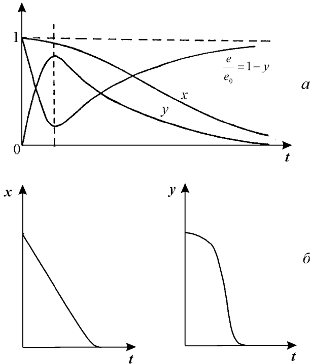
Рис. 6.3. Кинетика изменения безразмерных переменных в уравнении Михаэлиса–Ментен. a — с учетом области переходных процессов на малых временах (полная система 6.11). б — без учета области переходных процессов (редуцированная система 6.12).
