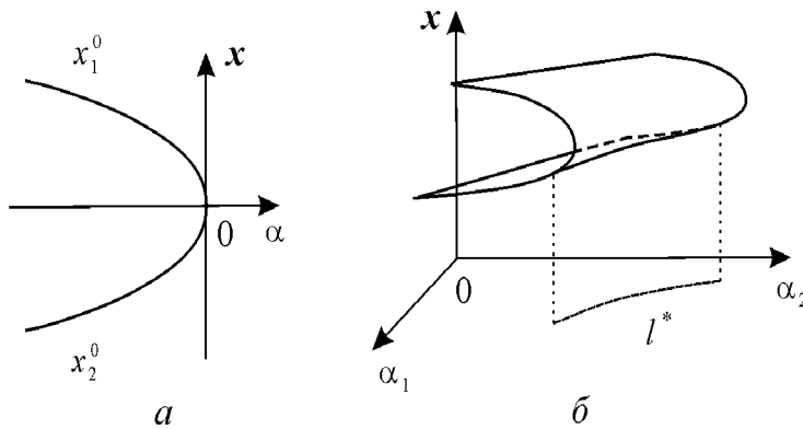
Рис. 6.6. Фазопараметрическая диаграмма бифуркации седло-узел: a — с одним управляющим параметром. При \alpha > 0 в системе нет устойчивых равновесий, при \alpha < 0 в системе два равновесия, устойчивое и неустойчивое, b — бифуркации седло-узел с двумя управляющими параметрами (катастрофа типа складка). l^* — линия бифуркации на плоскости параметров \alpha_1, \alpha_2 .
