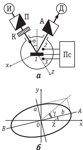
Рис. 7.20. Принципиальная схема эллипсометрического метода (а) и проекция на плоскость xу траектории, описываемой концом вектора электрического поля падающего света (б):
