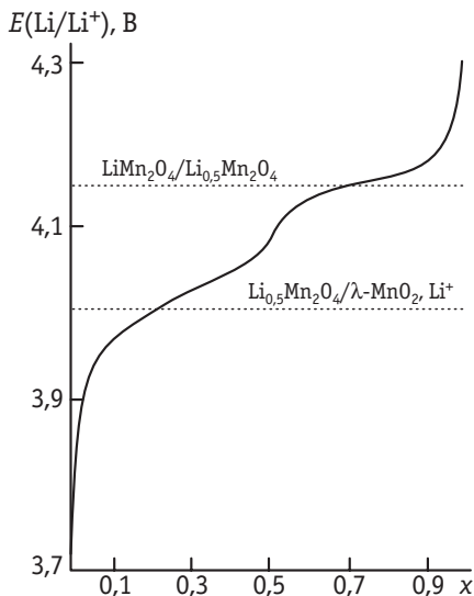
Рис. 10.20. Гальваностатическая кривая заряжения литий-марганцевой шпинели в растворе 1 М \text{LiAsF}_6 (растворитель — смесь 1:3 этиленкарбоната и диметилкарбоната). Пунктиром обозначены потенциалы двух равновесий с участием твердых фаз. Площадки потенциала отвечают сосуществованию двух фаз, участвующих в этих равновесиях
