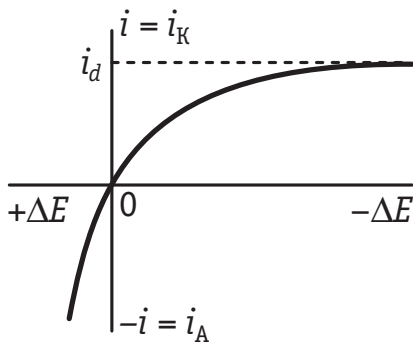
Рис. 8.3. Зависимость тока от концентрационной поляризации при разряде ионов металла на одноименном металле
