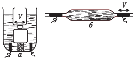
Рис. 5.3. Типы ячеек для измерения чисел переноса в расплавах (пояснение в тексте)
