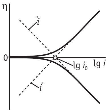
Рис. 9.3. Поляризационная кривая стадии переноса заряда при g_0 = \text{const} , g_R = \text{const} , \alpha = 0,5 и \psi_1 = \text{const} в полулогарифмических координатах
