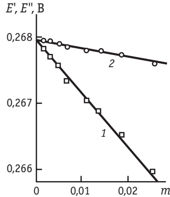
Рис. 6.9. Уточненный графический метод определения стандартного потенциала хлорсеребряного электрода по измерениям ЭДС:
