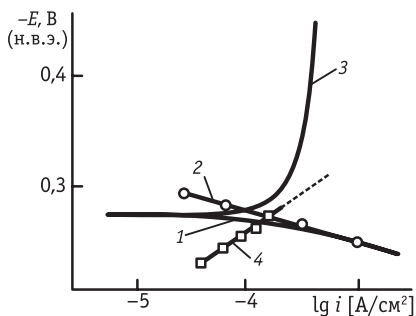
Рис. 10.7. Поляризационные кривые для амальгамы индия в растворе In(ClO_4)_3 + NaClO_4 :
