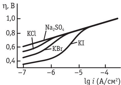
Рис. 9.17. Зависимость перенапряжения водорода от плотности тока на ртути в подкисленных 1 М растворах KCl, KBr, KI и 0,5 М растворе \text{Na}_2\text{SO}_4
