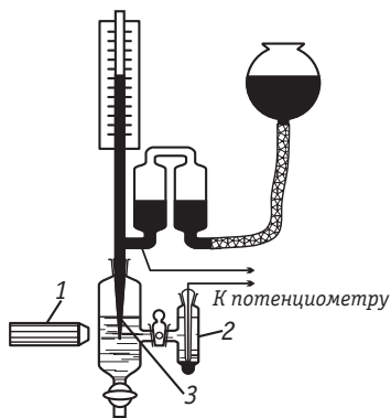
Рис. 7.6. Упрощенная схема капиллярного электрометра Гуи:
