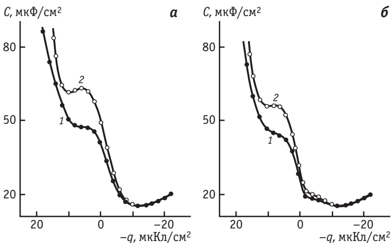
Рис. 7.34. Кривые дифференциальной емкости ртутного электрода в 0,1 М (а) и 0,01 М (б) водных растворах КВг:
