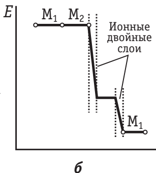
Рис. 7.26. Локализация разности потенциалов в правильно разомкнутой электрохимической цепи M_1 | M_2 | \text{электролит} | M_1 :
