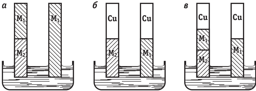
Рис. 6.2. Эквивалентные правильно разомкнутые электрохимические цепи. Пояснение в тексте
