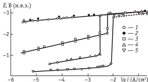
Рис. 9.24. Катодные поляризационные кривые для растворов различных солей в гексаметилфосфортриамиде:
