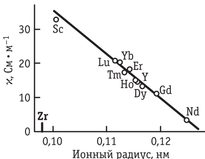
Рис. 5.12. Зависимость удельной электропроводности твердого электролита состава 0,91 \text{ ZrO}_2 \cdot 0,09 \text{ M}_2\text{O}_3 от ионного радиуса катиона редкоземельного металла при температуре 1000 °С
