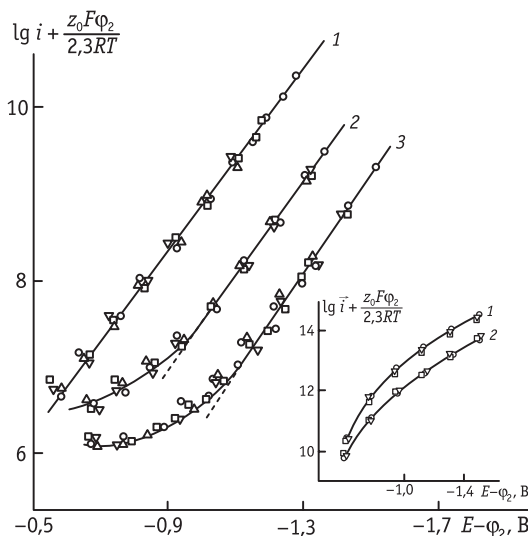
Рис. 9.20. Исправленные тафельские зависимости, построенные по полярографическим данным для растворов 5 \cdot 10^{-4} М \text{M}_2\text{S}_2\text{O}_8 с добавками хлоридов МСl:
