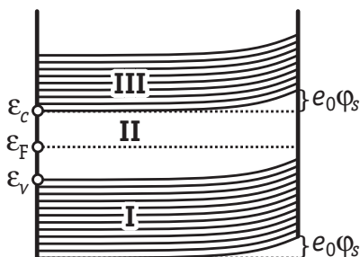
Рис. 9.40. Энергетические зоны полупроводникового электрода:
