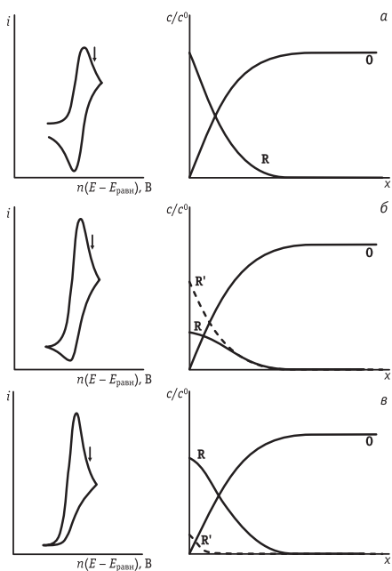
Рис. 10.5. Циклические вольтамперограммы, отвечающие реакции O + ne^- \rightleftharpoons R (а) и (10.2.Г) (б, в), и стабилизированное распределение концентраций O и R в приэлектродном слое для момента времени, обозначенного стрелкой:
