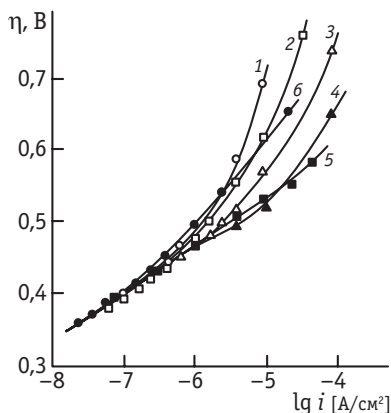
Рис. 9.39. Перенапряжение выделения водорода на ртути в подкисленных растворах солей:
