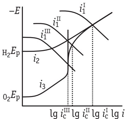
Рис. 10.15. Поляризационные кривые анодного растворения металлов ( i_1^I, i_1^{II}, i_1^{III} ), выделения водорода ( i_2 ) и восстановления кислорода ( i_3 ); i_c^I, i_c^{II}, i_c^{III} — токи саморастворения соответствующих металлов
