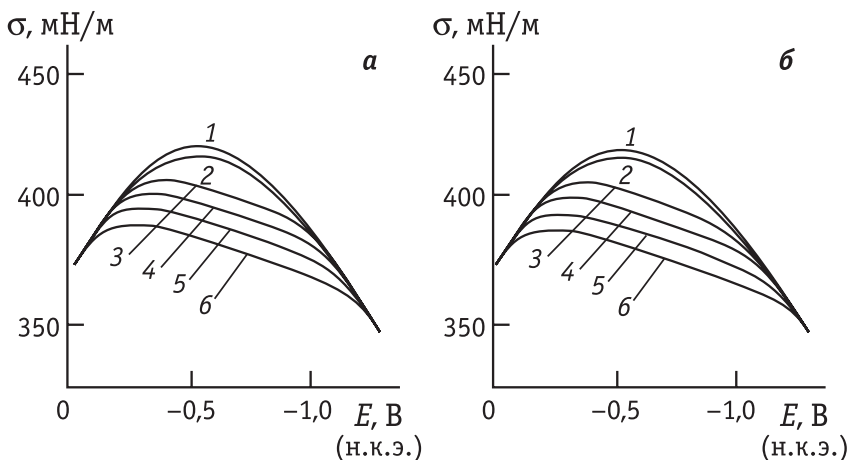
Рис. 7.40. Сопоставление экспериментальных (а) и рассчитанных по уравнению (7.14.27) (б) электрокапиллярных кривых для системы Hg/(1 М NaCl + x М трет -C 5 H 11 ОН) при x , равном: 0 (1); 0,01 (2); 0,05 (3); 0,1 (4); 0,2 (5) и 0,4 (6)
