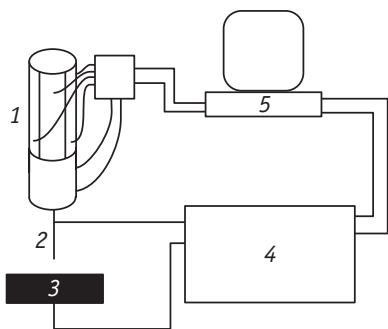
Рис. 7.22. Принципиальная схема сканирующего туннельного микроскопа (пояснения в тексте)
