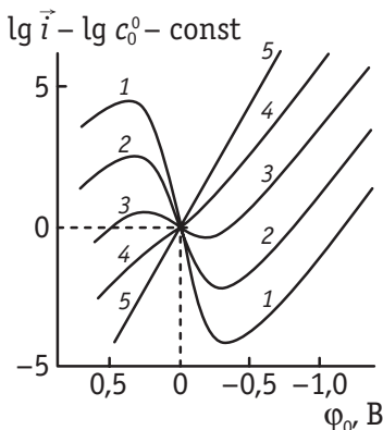
Рис. 9.4. Поляризационные кривые, рассчитанные по уравнению теории замедленного разряда при z_0 = 2 , \alpha n = 0,5 и \psi_1 = \psi_0 на ртутном электроде в растворах NaF:
