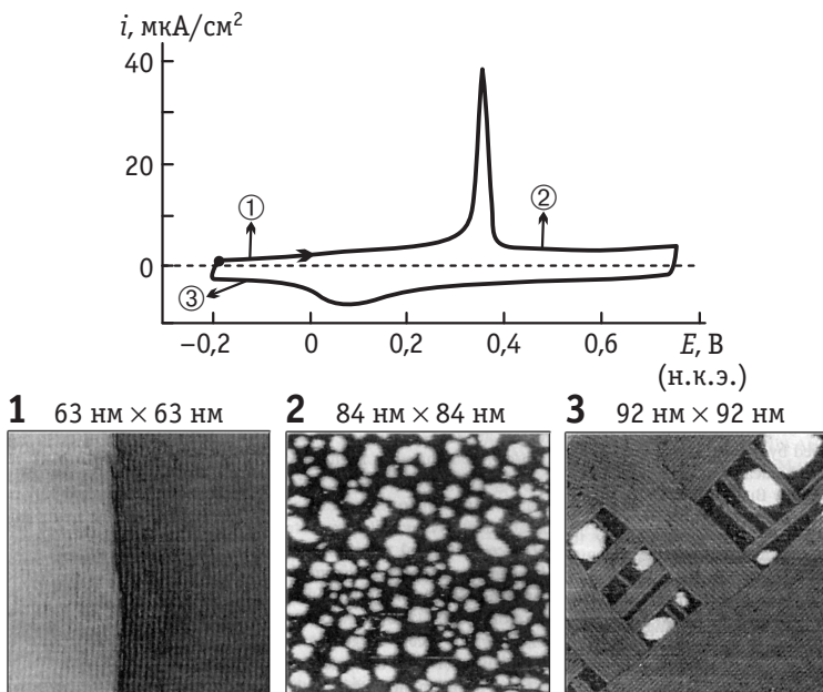
Рис. 7.25. Вольтамперограмма монокристаллического электрода Au(100) и туннельно-микроскопические изображения поверхности, зарегистрированные в разных областях потенциалов в ходе электрохимически индуцированной реконструкции
