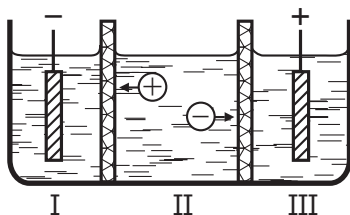
Рис. 4.5. Схема определения чисел переноса по методу Гитторфа
