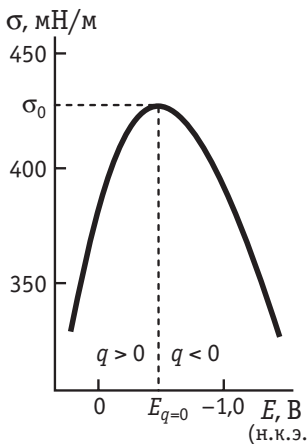
Рис. 7.7. Электрокапиллярная кривая ртутного электрода в 0,5 М растворе \text{Na}_2\text{SO}_4
