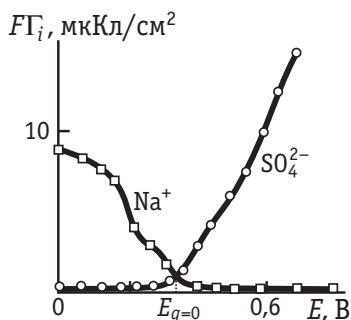
Рис. 7.5. Зависимость адсорбции ионов \text{Na}^+ и \text{SO}_4^{2-} от потенциала платинированного платинового электрода в растворе 5 \cdot 10^{-4} \text{ М H}_2\text{SO}_4 + 1,5 \cdot 10^{-3} \text{ М Na}_2\text{SO}_4 по данным адсорбционного радио-химического метода
