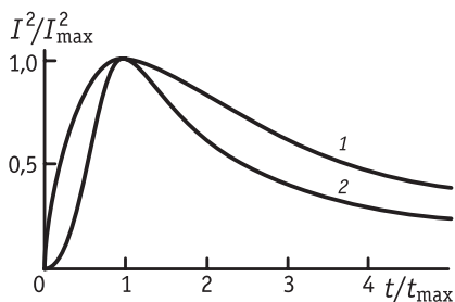
Рис. 10.19. Транзистенты тока в приведенных координатах:
