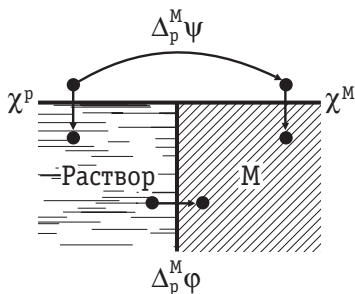
Рис. 7.28. Скачки потенциала на границе раствор/металл
