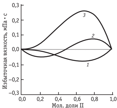
Рис. 5.9. Избыточная вязкость при 1100\text{ K} для систем I — II: \text{KCl} - \text{KBF}_4 (1), \text{KCl} - \text{K}_2\text{TiF}_6 (2), \text{KBF}_4 - \text{K}_2\text{TiF}_6 (3)
