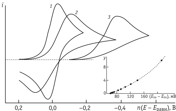
Рис. 9.14. Циклические вольтамперограммы, рассчитанные для скорости развертки 0,1 В/с, D = 10^{-5} см 2 /с и констант скорости k_s :
