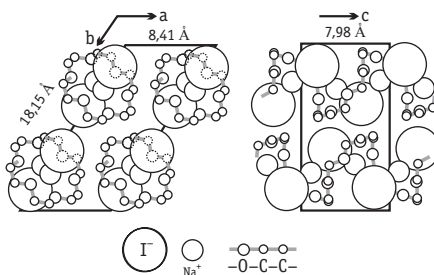
Рис. 5.17. Кристаллическая структура ТПЭ \text{NaI} \cdot (\text{ПЭО})_3
