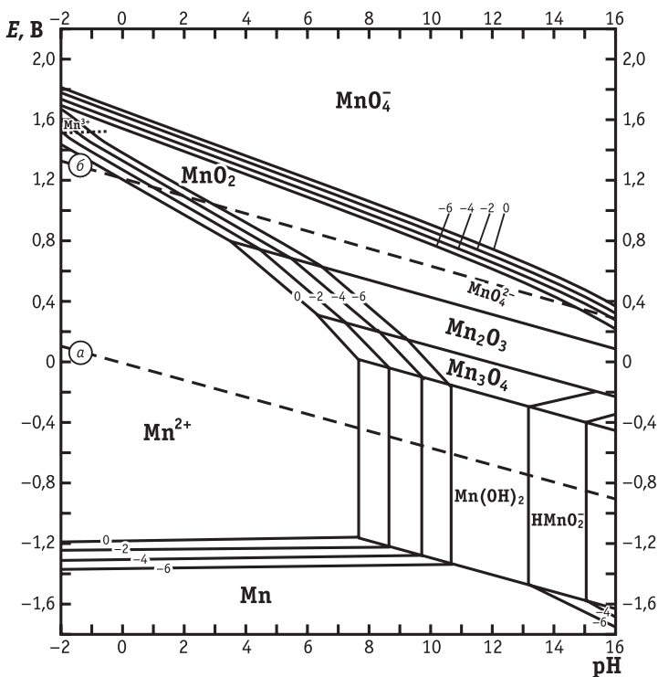
Рис. 6.4. Диаграмма E - \text{pH} для системы марганец — вода при 25^\circ\text{C}
