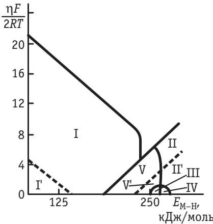
Рис. 10.11. Области с различными механизмами выделения водорода:
