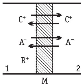
Рис. 6.10. Граница двух растворов CA + RA (1) и CA (2), разделенных полупроницаемой мембраной М
