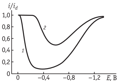
Рис. 9.22. Зависимости от потенциала «смешанного» тока, рассчитанные с точностью до постоянного множителя из поляризационных кривых (1 и 2 соответственно) стадии переноса заряда, приведенных на рис. 9.21, и предельного диффузионного тока i_d^{(0)} = 1 усл. ед.
