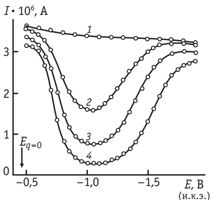
Рис. 9.18. Полярограммы, измеренные на ртутном капающем электроде в растворах 5 \cdot 10^{-4} М K_2S_2O_8 с добавками KCl: 1 — 10^{-1} М; 2 — 10^{-2} М; 3 — 5 \cdot 10^{-3} М; 4 — 2 \cdot 10^{-3} М
