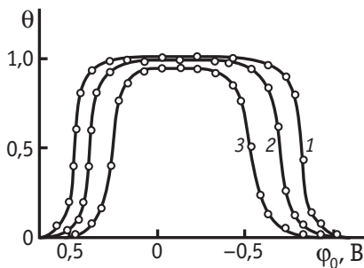
Рис. 7.37. Зависимость заполнения поверхности органическим веществом от потенциала электрода для системы Hg/(0,9 М NaF + x М трет -C 5 H 11 OH) при x , равном 0,3 (1), 0,1 (2), 0,03 (3)
