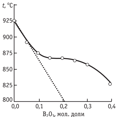
Рис. 5.6. Кривые ликвидуса \text{K}_2\text{MoO}_4 в системе \text{K}_2\text{MoO}_4 + \text{B}_2\text{O}_3
