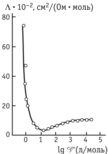
Рис. 4.14. Зависимость эквивалентной электропроводности \Lambda от разведения V для раствора металлического натрия в жидком аммиаке при -33,5^\circ\text{C}
