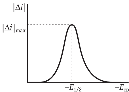
Рис.8.11. Полярограмма на переменном токе, рассчитанная по формулам (8.6.9) и (8.6.7)
