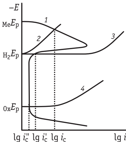
Рис. 10.18. Саморастворение металла при пассивации:
