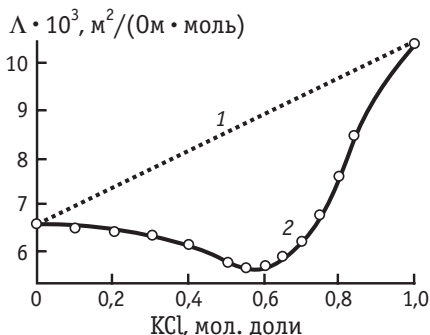
Рис. 5.8. Зависимость эквивалентной электропроводности от состава расплава в смеси \text{CdCl}_2 — \text{KCl} при 720^\circ\text{C} : 1 — при строгой аддитивности электропроводности; 2 — опытные данные
