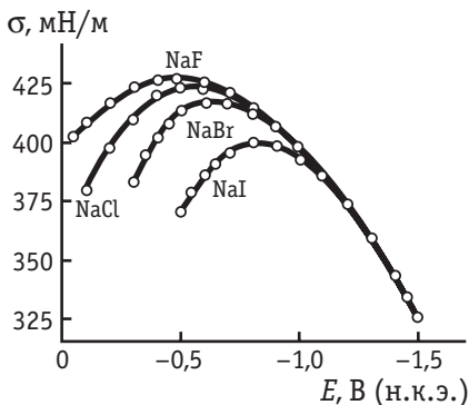
Рис. 7.10. Электрокапиллярные кривые ртутного электрода в 0,9 М растворах галогенидов натрия
