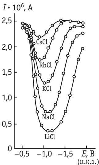
Рис. 9.19. Полярограммы, измеренные на ртутном капельном электроде в растворах 5 \cdot 10^{-4} М \text{K}_2\text{S}_2\text{O}_8 с добавками 0,01 М солей щелочных металлов
