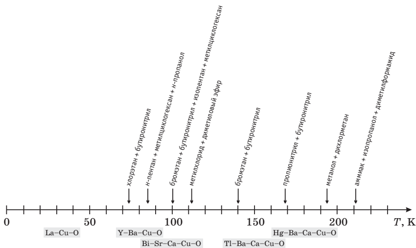
Рис. 2.7. Низкотемпературные квазижидкие системы, разработанные в связи с задачами электрохимии купратных сверхпроводников A_xB_yCuO_z ( A = Ba, Sr, Ca ; B = La, Y, Bi, Tl, Hg )
