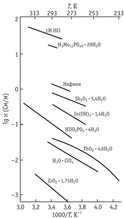
Рис. 5.20. Зависимости проводимости \kappa некоторых кристаллогидратов от температуры. Для сравнения приведены данные для водного раствора 1 М HCl и нафийона
