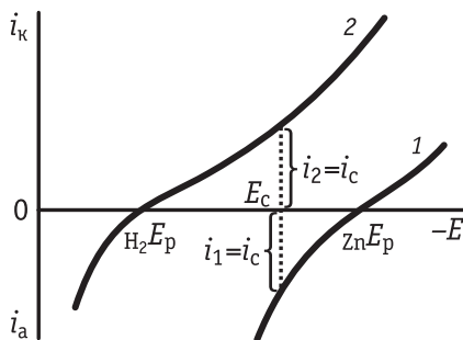
Рис. 10.12. Поляризационные кривые разряда и ионизации цинка (1) и водорода (2)
