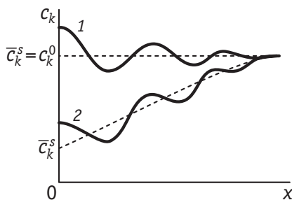
Рис. 8.10. Зависимость концентрации c_k реагирующего вещества k от расстояния до поверхности электрода x в условиях, когда заданный потенциал электрода подчиняется уравнению (8.6.1):
