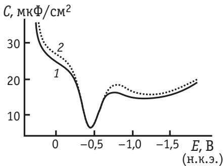
Рис. 7.32. Сопоставление экспериментальной (1) и теоретически рассчитанной (2) кривых емкости ртутного электрода в 0,001 М водном растворе NaF
