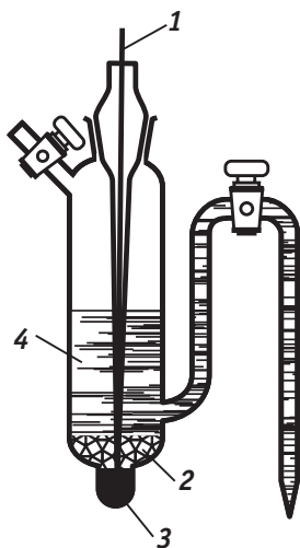
Рис. 6.5. Схема каломельного электрода:
