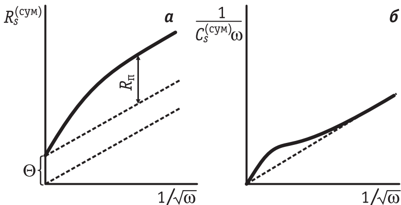
Рис. 10.2. Зависимость суммарных омической (а) и емкостной (б) компонент импеданса, измеренных по последовательной схеме замещения, от 1/\sqrt{\omega} при наличии стадий диффузии, переноса заряда и гетерогенной химической реакции. R_\pi = RT / (n^2 F^2 \bar{\Gamma}_R \kappa) . Пунктирная линия на рис. «б» и нижняя пунктирная линия на рис. «а» отвечают только стадиям диффузии, а верхняя пунктирная линия на рис. «а» — стадиям диффузии и переноса заряда в отсутствие химической реакции
