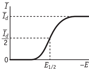
Рис. 8.8. Идеальная форма полярограммы:
