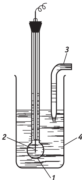
Рис. 6.11. Стекланный электрод:
