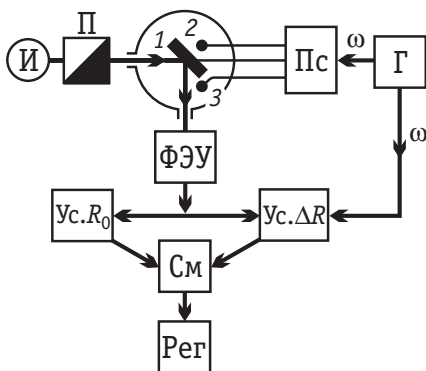
Рис. 7.21. Принципиальная схема метода модуляционной спектроскопии отражения:
