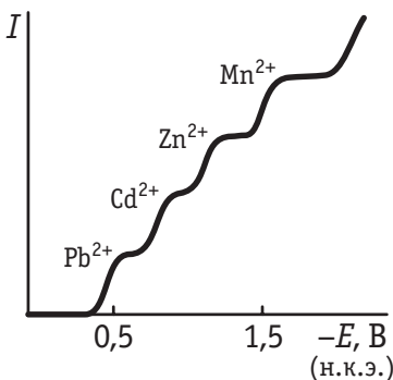
Рис. 8.9. Полярограмма раствора, содержащего 5 \cdot 10^{-4} М \text{Pb}^{2+} , \text{Cd}^{2+} , \text{Zn}^{2+} , \text{Mn}^{2+} в присутствии 1 М \text{KCl}
