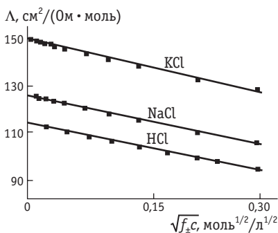
Рис. 4.11. Зависимость молярной электропроводности водных растворов хлоридов от корня квадратного из средней активности
