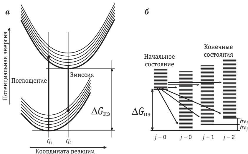
Рис. 9.26. Оптические переходы в инвертированной маркусовской области: a — электронные термы; б — схематическое изображение колебательных мод (горизонтальными стрелками изображены безызлучательные переходы, наклонными — флуоресценция)
