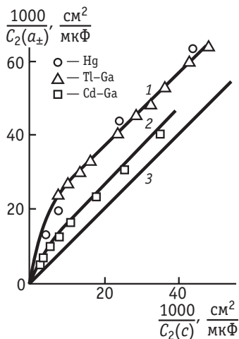
Рис. 7.33. Зависимости обратной емкости диффузного слоя C_2(a_{\pm}) , рассчитанной по модели Гонзалеса — Санса, от обратной емкости диффузного слоя C_2(c) , рассчитанной по модели Гуи — Чапмена — Грэма, для растворов \text{La}_2(\text{SO}_4)_3 (1) и \text{Na}_2\text{SO}_4 (2). Прямая 3 с единичным наклоном проведена через начало координат. Точки — опытные данные для Hg и сплавов Tl-Ga и Cd-Ga
