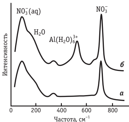
Рис. 1.3. Рамановские спектры водного раствора 3 \text{ М Al}(\text{NO}_3)_3 : а — в неполяризованном, б — в поляризованном свете
