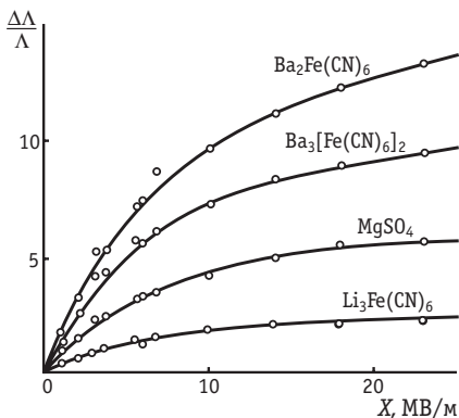
Рис. 4.10. Эффект Вина для некоторых сильных электролитов
