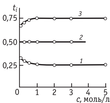
Рис. 4.7. Зависимость чисел переноса t_i от концентрации водных растворов электролитов с при 18 °С: 1 — t_+ в растворе LiCl; 2 — t_+ в растворе KCl; 3 — t_- в растворе LiCl
