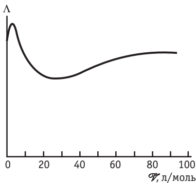
Рис. 4.12. Схематический вид зависимости эквивалентной электропроводности \Lambda от разведения c в неводных растворителях
