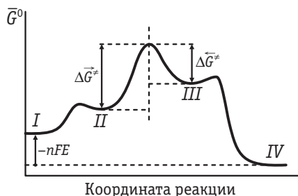
Рис. 9.1. Зависимость электрохимической стандартной свободной энергии системы \bar{G}^0 от пути реакции O + ne^- \rightleftharpoons R
