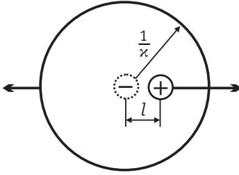
Рис. 4.8. Схема асимметрии ионной атмосферы для оценки релаксационного эффекта
