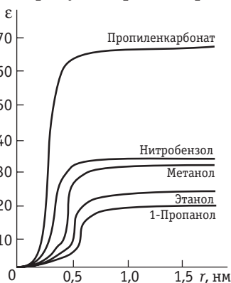
Рис. 3.6. Зависимость диэлектрической проницаемости \epsilon от расстояния, отсчитываемого от центра сольватируемого иона
