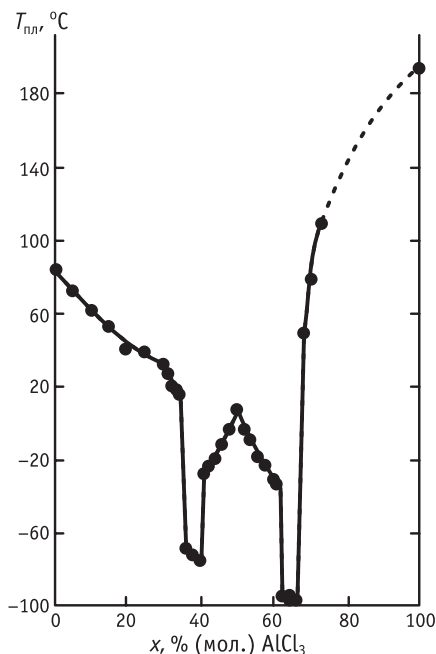
Рис. 5.1. Зависимость температуры плавления смеси \text{AlCl}_3 — хлорид этилметилимидазолия от ее состава
