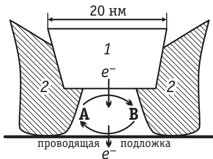
Рис. 8.18. Микроочаг для регистрации электрохимических превращений единичной молекулы:
