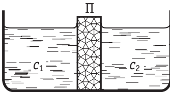
Рис. 4.1. Контакт двух растворов различной концентрации, который приводит к возникновению диффузионного потенциала (П — пористая перегородка)
