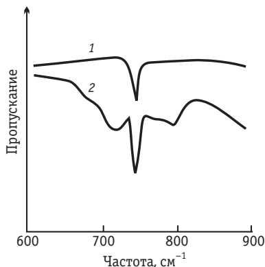
Рис. 5.5. ИК-спектр застеклованных \text{KBF}_4 (1) и \text{KBF}_4 + \text{KCl} (2)
