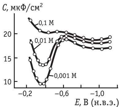
Рис. 7.13. Кривые емкости двойного слоя висмутового электрода в водных растворах КФ различной концентрации
