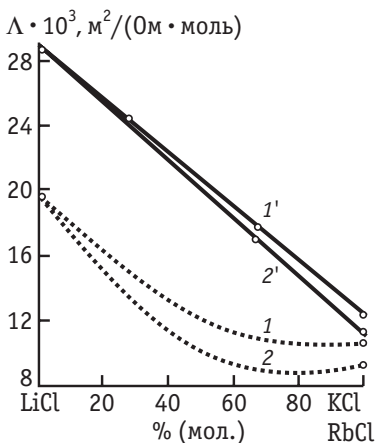
Рис. 5.7. Изотермы предельной высоковольтной (1', 2') и низковольтной (1, 2) мольной электропроводности бинарных смесей LiCl - KCl (1, 1') и LiCl - RbCl (2, 2') при 1073 К
