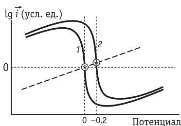
Рис. 9.21. Поляризационные кривые электровосстановления анионов ( z_0 = -2 , \alpha = 0,3 ), рассчитанные по уравнению (9.6.7) для двух металлов M_1 (1) и M_2 (2) \Delta E_{q=0} = 0,2 В в предположении, что \psi_1 = \frac{2RT}{F} \cdot \text{arcsh} \left( \frac{q}{2A\sqrt{c}} \right) ; c = 0,001 М; q = C(E - E_{q=0}) ; C = 23,5 мкФ/см 2 . Для металла M_1 принято \ln c_0 + \text{const} = 0 и E_{q=0}^{(M_1)} = 0
