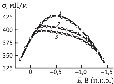
Рис. 7.11. Электрокапиллярные кривые ртутного электрода в 0,5 М растворе \text{Na}_2\text{SO}_4 (1), а также с добавками 0,1 М n\text{-C}_4\text{H}_9\text{OH} (2) и 0,2 М n\text{-C}_4\text{H}_9\text{OH} (3)
