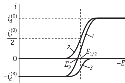
Рис. 8.2. Зависимости тока от потенциала:
