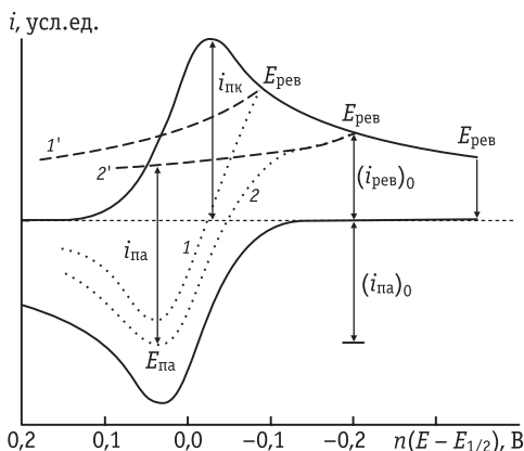
Рис. 8.13. Циклические вольтаграммы, измеренные в присутствии в растворе окисленной формы O (при отсутствии продукта восстановления R в объеме раствора). Точками показаны кривые 1, 2 , полученные в случае изменения направления развертки при разных потенциалах E_{\text{рев}} . Пунктиром обозначены линии отсчета (кривые 1' и 2' ), отвечающие изменению катодной составляющей тока в ходе анодной развертки и относящиеся к кривым 1 и 2 соответственно. Нижняя (сплошная) кривая анодного хода отвечает выдержке при наиболее отрицательном значении E_{\text{рев}} до достижения нулевого тока
