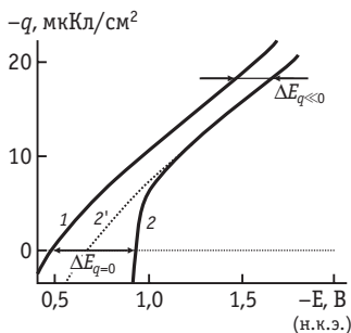
Рис. 7.29. Кривые заряда поверхности ртутного (1) и галлиевого (2) электродов в водном растворе 0,1 M \text{Na}_2\text{SO}_4 . Пунктирная кривая 2' проведена симбатно кривой 1
