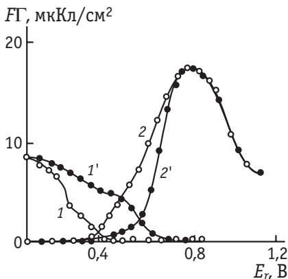
Рис. 7.41. Зависимость адсорбции катионов \text{Na}^+ (1, 1') и анионов \text{SO}_4^{2-} (2, 2') на платинированной платине в растворе 5 \cdot 10^{-4} М \text{H}_2\text{SO}_4 + 1,5 \cdot 10^{-4} М \text{Na}_2\text{SO}_4 при отсутствии (1, 2) и в присутствии (1', 2') адсорбированного метанола
