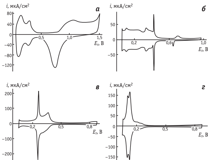
Рис. 7.17. Вольтамперограммы, измеренные в растворе 0,5 М \text{H}_2\text{SO}_4 при скорости развертки потенциала 50 мВ/с на поликристаллической платине (а) и отожженных гранях монокристалла платины (111) (б), (100) (в) и (110) (г). Потенциал E_r приведен в шкале обратимого водородного электрода (о. в. э.) в том же растворе
