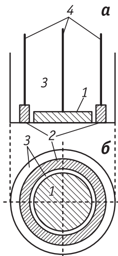
Рис. 8.5. Рабочая часть вращающегося дискового электрода с кольцом в разрезе (а) и с торца (б): 1 — диск; 2 — кольцо; 3 — тефлоновая оболочка; 4 — токоотводы
