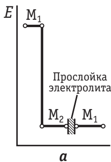
Рис. 7.26. Локализация разности потенциалов в правильно разомкнутой электрохимической цепи M_1 | M_2 | \text{электролит} | M_1 :
