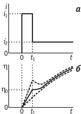
Рис. 9.9. Зависимость тока (а) и перенапряжения (б) от времени в двухимпульсном гальваностатическом методе
