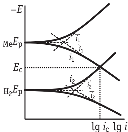
Рис. 10.13. Зависимость скоростей реакций разряда и ионизации металла ( \bar{i}_1 и \bar{i}_1 ) и водорода ( \bar{i}_2 и \bar{i}_2 ), а также суммарной скорости растворения металла ( i_1 ) и выделения водорода ( i_2 ) от потенциала
