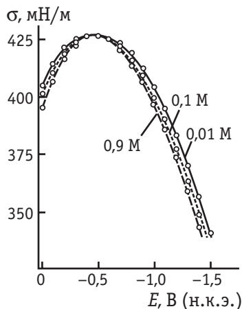
Рис. 7.8. Электрокапиллярные кривые ртутного электрода в водных растворах фторида натрия разной концентрации
