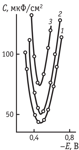
Рис. 7.42. Кривые дифференциальной емкости свинцового электрода в расплавах солей: NaCl при 820 °С (1), NaBr при 800 °С (2), NaI при 800 °С (3)
