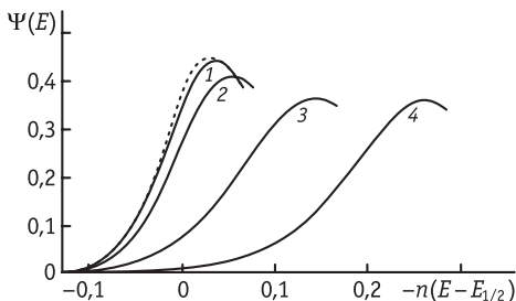
Рис. 9.13. Зависимость функции \Psi от потенциала электрода, отсчитанного от потенциала полувольны, для \alpha = 0,5 и \Lambda = 10 (1), 1 (2), 0,1 (3), 0,01 (4). Пунктир — вольтамперограмма обратимого процесса
