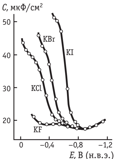
Рис. 7.14. Кривые емкости двойного слоя висмутового электрода в 0,1 М водных растворах галогенидов калия
