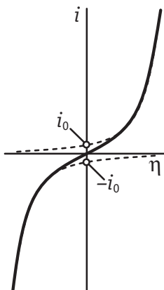
Рис. 9.2. Поляризационная кривая стадии переноса заряда при g_0 = \text{const} , g_R = \text{const} , \alpha = 0,5 и \psi_1 = \text{const}
