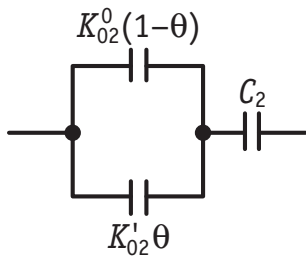
Рис. 7.36. Эквивалентная электрическая схема модели Алексеева — Попова — Колотыркина
