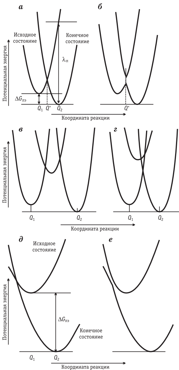
Рис.9.25. Схематическое изображение электронных термов для реакций одноэлектронного (а, б, д, е) и двухэлектронного (в, г) процессов в случае неадиабатического (а, в, г, д) и адиабатического (б, е) переноса в нормальной (а-г) и инвертированной (д, е) маркусовских областях
