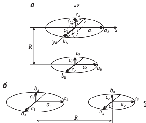
Рис. 9.27. Возможные расположения реагентов в модели проводящих эллипсоидов вращения
