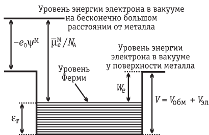
Рис. 7.30. Схема потенциального «металл-ящика» в модели «желе»
