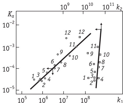
Рис. 4.17. Зависимость константы равновесия K_a от констант скорости диссоциации k_1 и рекомбинации k_2 слабых кислот в присутствии раствора 1 М LiCl при 20 °С:
