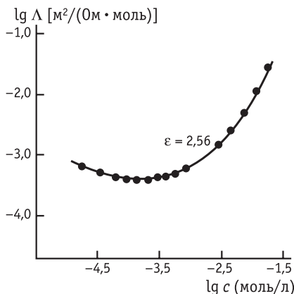
Рис. 4.13. Зависимость эквивалентной электропроводности \Lambda раствора нитрата тетраизоамиламмония в водно-диоксановой смеси от концентрации c
