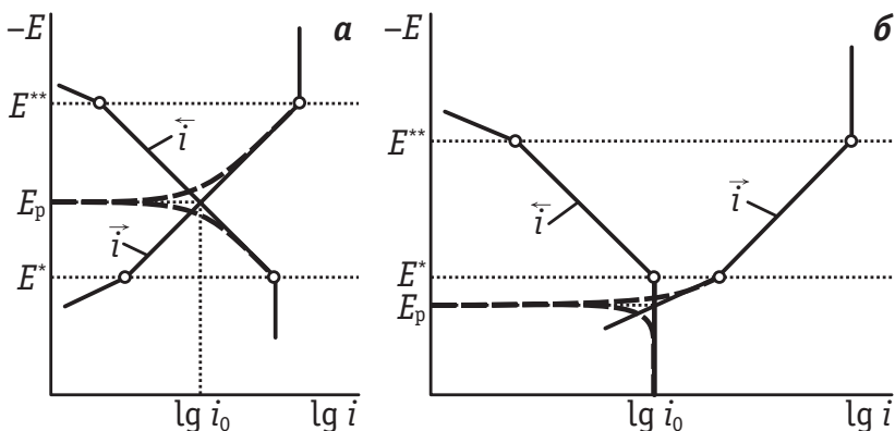
Рис. 9.38. Поляризационные кривые прямого ( \vec{i} ) и обратного ( \overleftarrow{i} ) токов в области безбарьерного ( E > E^* ), обычного ( E^* > E > E^{**} ) и безактивационного ( E < E^{**} ) разряда (упрощенная схема):
