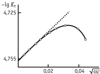
Рис. 3.5. Зависимость константы диссоциации уксусной кислоты от концентрации
