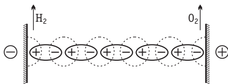
Рис. 1.1. Механизм электропроводности по Гроттусу
