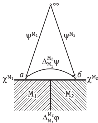
Рис. 7.27. Скачки потенциала на границе двух металлов
