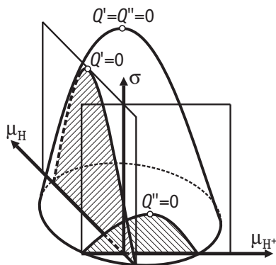
Рис. 7.19. Электрокапиллярные кривые первого и второго рода водородного электрода, представленные в виде сечений поверхности \sigma плоскостями \mu_{\text{H}^+} = \text{const} и \mu_{\text{H}} = \text{const}
