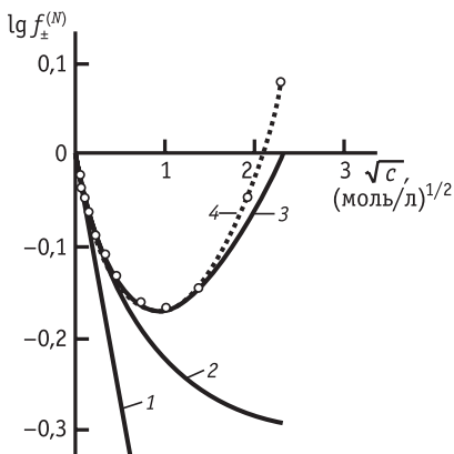
Рис. 3.4. Зависимость среднего коэффициента активности от концентрации в водном растворе NaCl:
