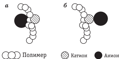
Рис. 5.18. Сольватно-разделенные (а) и сольватно-неразделенные (б) ионные пары в ТПЭ
