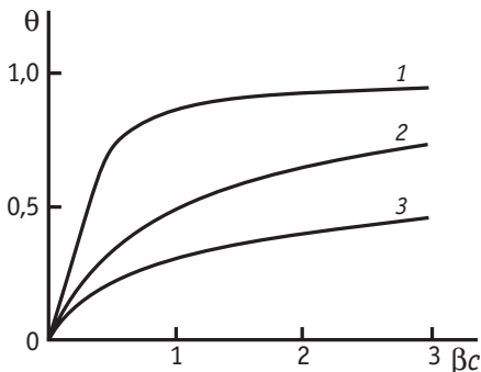
Рис. 7.39. Изотермы адсорбции, рассчитанные по уравнению (7.14.26) при различных значениях аттракционной постоянной a : 1,15 (1), 0 (2), -1,15 (3)
