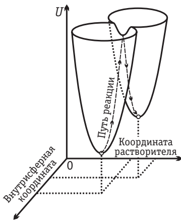
Рис. 9.31. Зависимости электронных термов начального и конечного состояний от координат растворителя и растяжения химических связей с низкими частотами собственных колебаний
