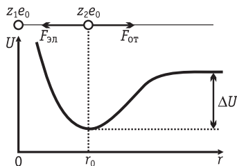
Рис. 2.1. К расчету энергии взаимодействия двух ионов
