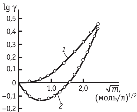
Рис. 3.1. Зависимость коэффициента активности тростникового сахара (1) и хлорида лития (2) от их концентрации в водном растворе
