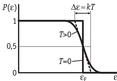
Рис. 9.35. Распределение электронов по энергиям в соответствии со статистикой Ферми — Дирака
