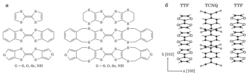
Рис. 5.21. «Органические металлы»:
