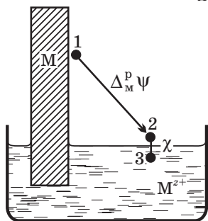
Рис. 2.3. Схема для расчета реальной энергии сольватации иона
