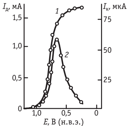
Рис. 10.9. Зависимости тока на диске I_d (1) и на кольце I_k (2) от потенциала диска при восстановлении кислорода на платине в 1 М КОН. Скорость вращения электрода 3800 об/мин
