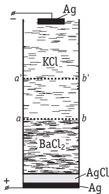
Рис. 4.6. Схема определения чисел переноса методом движущейся границы
