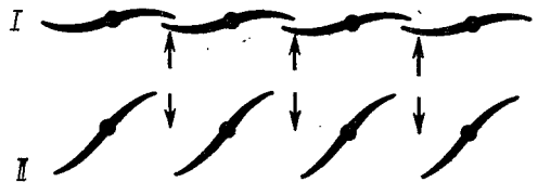
Рис. 40. Схема положения маховых перьев (в поперечном разрезе) и направление сопротивления воздуха (стрелки) при опускании крыла (I) и при его подъеме (II) (по Гессе)
