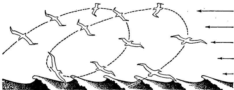
Рис. 47. Схема динамического парения (по Питерсону). Длина стрелок показывает относительную скорость ветра на разной высоте
