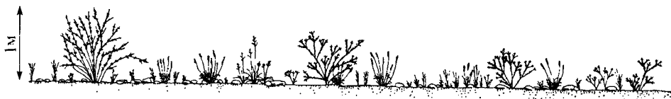
Рис. 292. Профиль тропической кустарниковой пустыни (по Г. Вальтеру, 1962)
