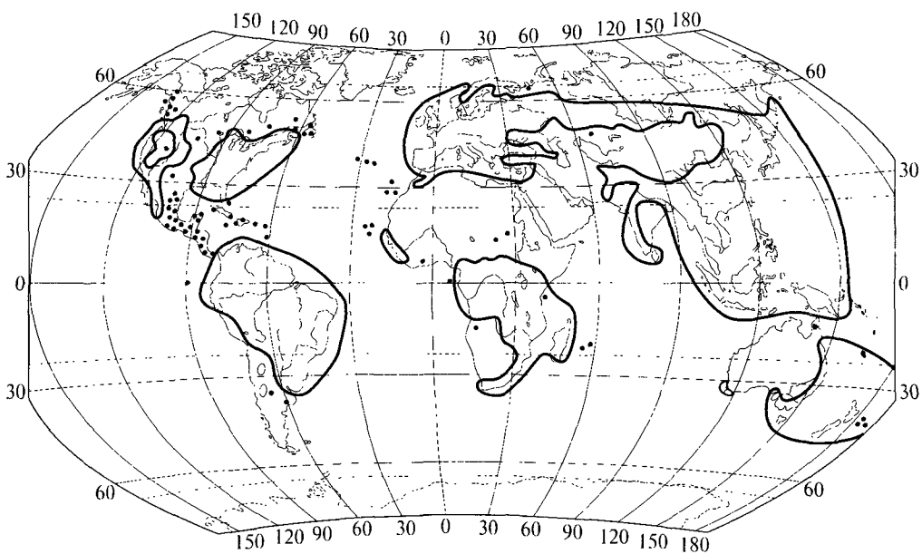
Рис. 279. Космополитический ареал орляка обыкновенного ( Pteridium aquilinum ) (по Ф. Фукареку и др., 1982).
