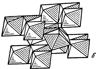
Рис. 99. Кристаллическая структура колумбита (а) и \alpha -PbO 2 (б)
