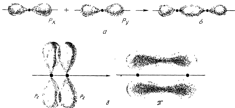
Рис. 15. Схема перекрывания и распределения валентных p -электронов: \alpha — образование \sigma -связи; \beta — боковое перекрывание двух p -орбиталей при образовании \pi -связи
