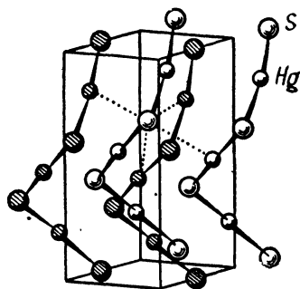
Рис. 101. Структура киновари \text{HgS}
