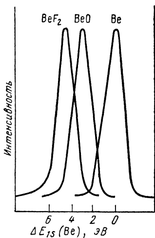
Рис. 52. Относительные положения 1s -уровня \text{Be} в металлическом \text{Be} , \text{BeO} и \text{BeF}_2
