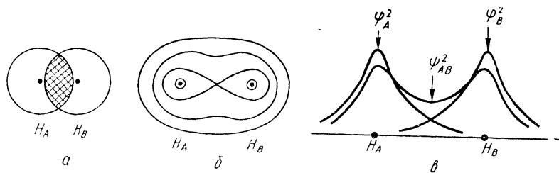
Рис. 14 Схема образования ковалентной связи между атомами водорода. а — перекрывание электронных оболочек; б — карта электронной плотности, в — сечение атомных ( \varphi_A^2 , \varphi_B^2 ) и молекулярной ( \psi_{AB}^2 ) электронных плотностей вдоль оси молекулы
