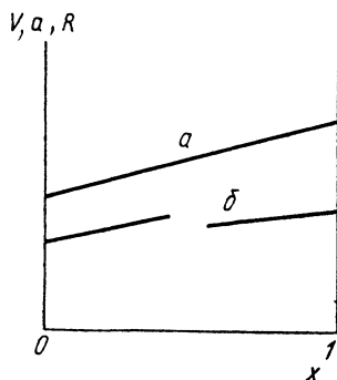
Рис. 108. Иллюстрация к правилам Ретгерса и Вегарда: a — изоморфизм, b — изодиморфизм
