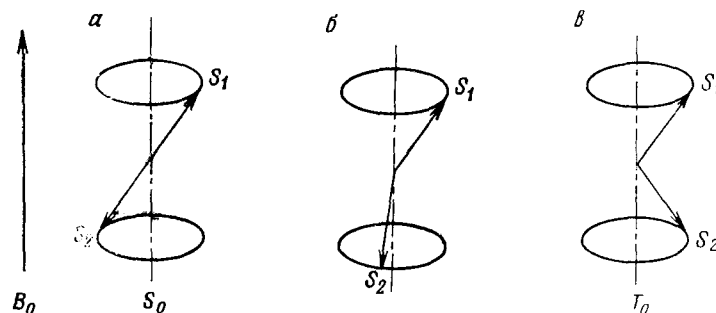
Рис. IX.28. Спиновые состояния радикальной пары в магнитном поле B_0 . а — синглетное состояние S_0 с суммарным спином, равным 0; фазовый угол равен 180^\circ ; б — различие в скоростях прецессии электронных спинов приводит к изменению фазового угла; в — триплетное состояние T_0 с суммарным спином, равным 1; фазовый угол составляет 0^\circ .
