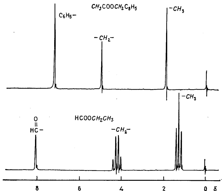
Рис. II. 11. Спектры ЯМР бензилацетата и этилформата.
