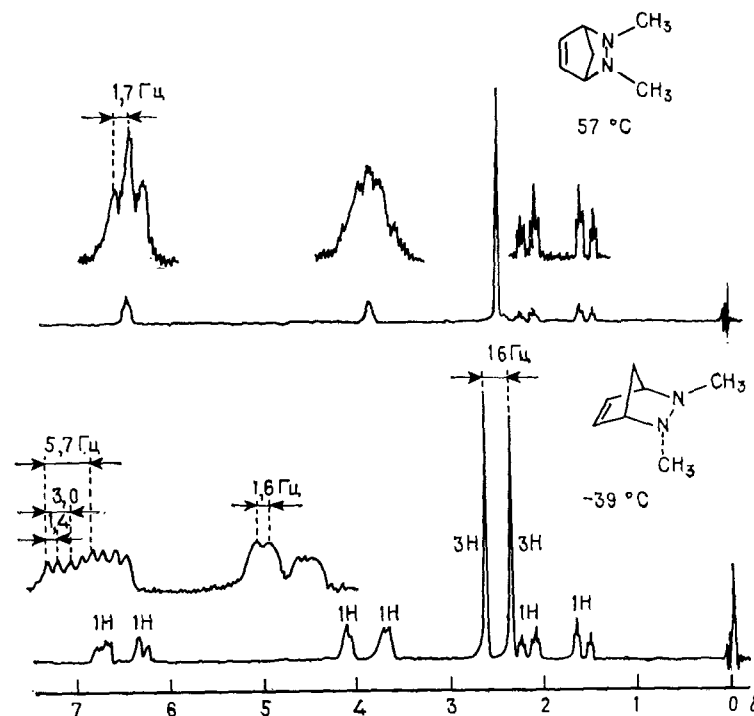
Рис. VIII.7. Температурная зависимость спектра ЯМР ^1\text{H} 2,3-диазабицикло[2.2.1]гептена-5 (147) (Андерсон, Лен [2]).
