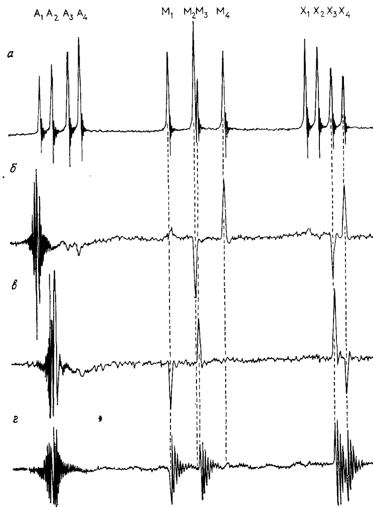
Рис. IX. 15. Спектр ЯМР ( a ), ИНДОФ-спектры ( b , v ) и осцилляции Торри ( z ) в системе AMX 2,3-дибромпропионовой кислоты (188).
