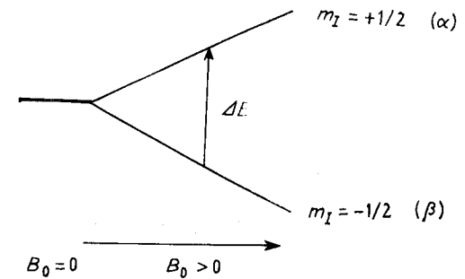
Рис. 1.2. Расщепление энергетических уровней протона в магнитном поле.
