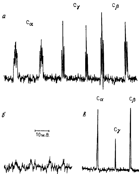
Рис. X. 6. Спектры ЯМР ^{13}\text{C} пиридина.
