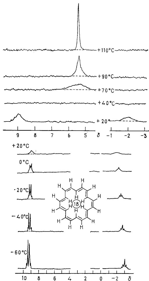
Рис. VIII. 11. Температурная зависимость спектра ЯМР [18]аннулена (3-изомер и сотр. [6]).
