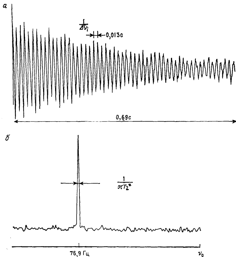
Рис. VII.18. Сигнал приемника, соответствующий одиночному сигналу ЯМР. a — во временном представлении как спад свободной индукции (ССИ); b — в частотном представлении в форме кривой Лоренца.
