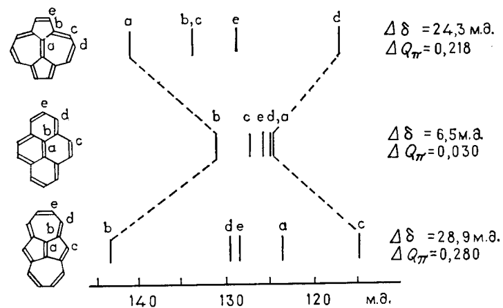
Рис. X.17. Химические сдвиги ^{13}\text{C} и разность зарядовой плотности в пирене и двух изомерных системах — дicyclopentaheptалене и дicyclopentaheptалене; значения \Delta Q_{\pi} рассчитаны методом ППДП/2 (Гюнтер, Шмиклер [12]).
