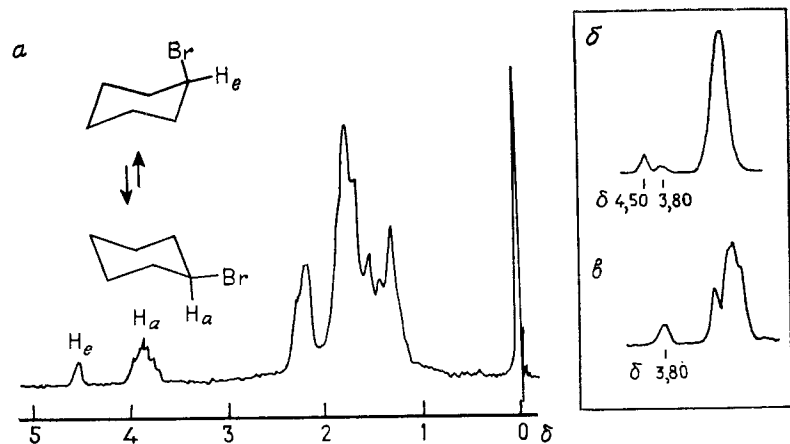
Рис. VIII.10. Спектры ЯМР монозамещенных циклогексанов. a — равновесная смесь аксиального и экваториального бромциклогексанов при -100^\circ\text{C} [4]; b — смесь аксиального и экваториального хлорциклогексанов при -150^\circ\text{C} (Дженсен, Башвиллер [5]); в — чистый экваториальный хлорциклогексан при -150^\circ\text{C} [5].
