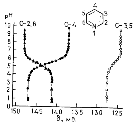
Рис. X.18. Зависимость положения сигналов в спектре пиридина от рН раствора (Брайтмаер, Спон [13]).
