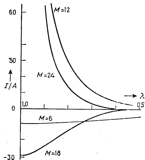
Рис. IV. 15. Интенсивность кольцевого тока I на единицу площади A в аннуленах в зависимости от параметра альтернирования \lambda . (Попл, Унч [4].)
