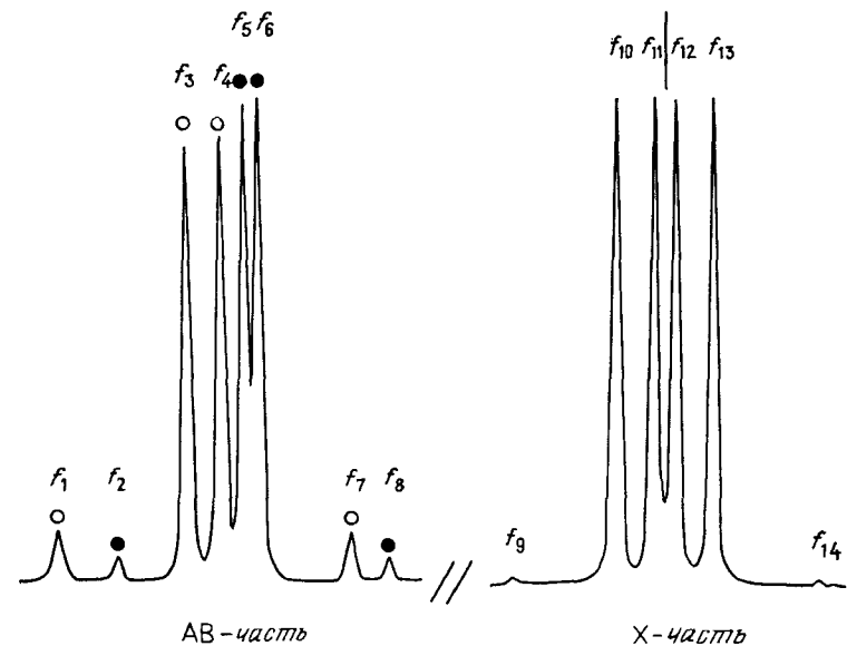
Рис. V. 10. Система АВХ с параметрами \nu_0\delta(AB) = 5,0 Гц, J_{AB} = 8 Гц, J_{AX} = 4,2 Гц и J_{BX} = 1,8 Гц. (Бови [1]). Подспектры аб-типа в АВ-части спектра обозначены незачерненными и зачерненными кружками. Используемые параметры относятся к 2-хлор-3-аминопиридину.
