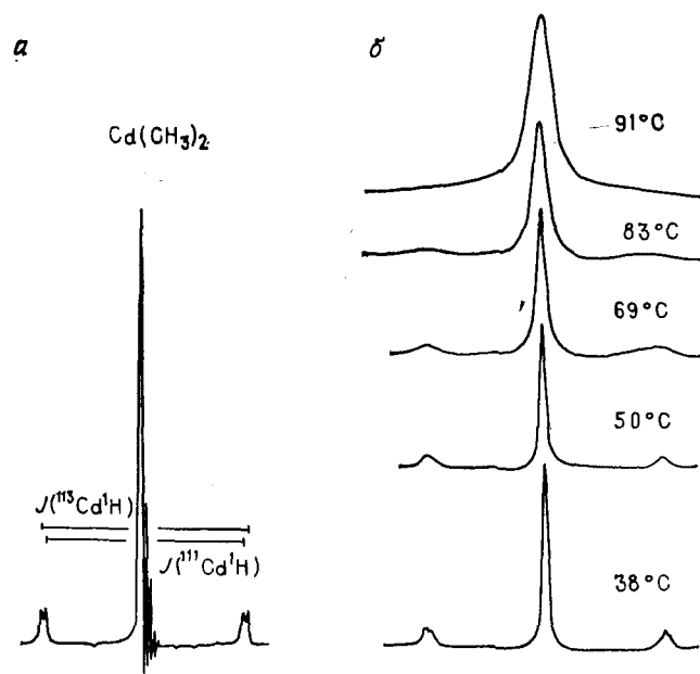
Рис. VIII. 21. \alpha — спектр ЯМР ^1\text{H} диметилкадмия в толуоле (Хэм, Моль [14]); \beta — температурная зависимость спектра ЯМР чистого диметилкадмия (Бремзер и сотр. [15]).
