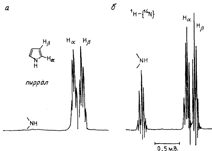
Рис. IX. 16. Спектр ЯМР ^1\text{H} пиррола [8]. а — без облучения; б — с облучением ядер ^{14}\text{N} .
