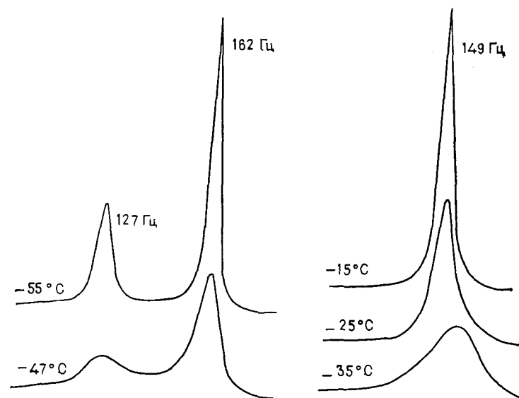
Рис. VIII. 20. Температурная зависимость ЯМР ^1\text{H} триметилалюминия в толуоле (Хэм, Моль [14]).
